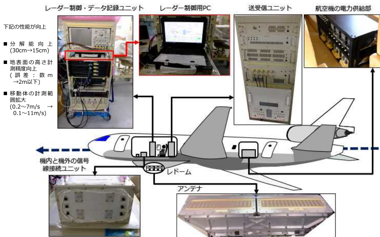
開発した超高精細航空機搭載合成開口レーダシステムの各機器
