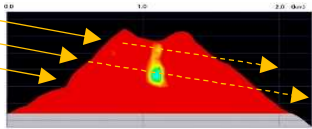
素粒子ミュオンを用いた火山透視技術の開発
