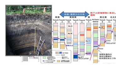
ボーリング、トレンチ調査、地表調査等による噴火履歴・推移の解明
