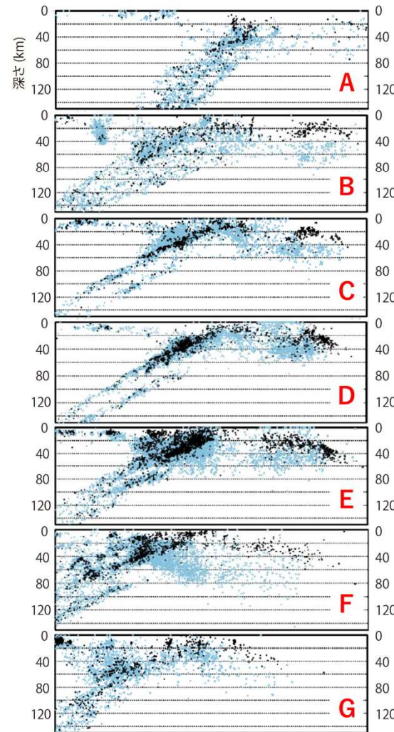
各矩形領域の断面図 (長辺投影)
