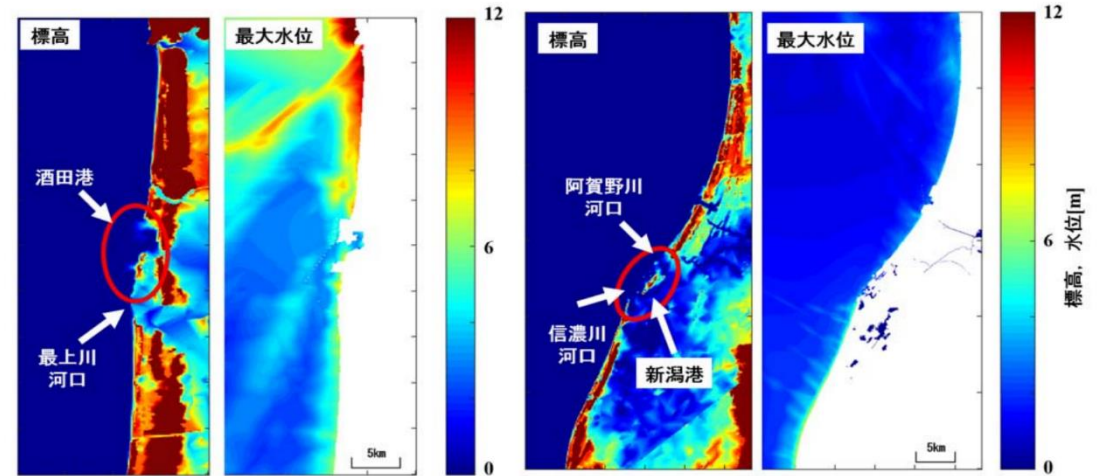
Web上で実装した高速津波計算システム
