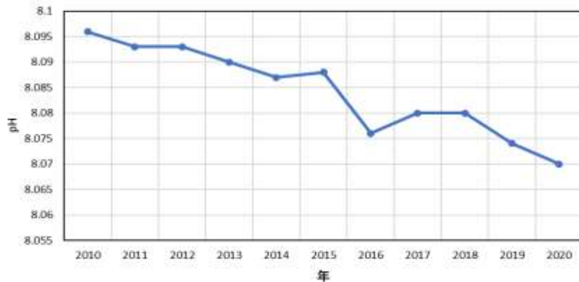
東経137度における平均pHの時間変化
