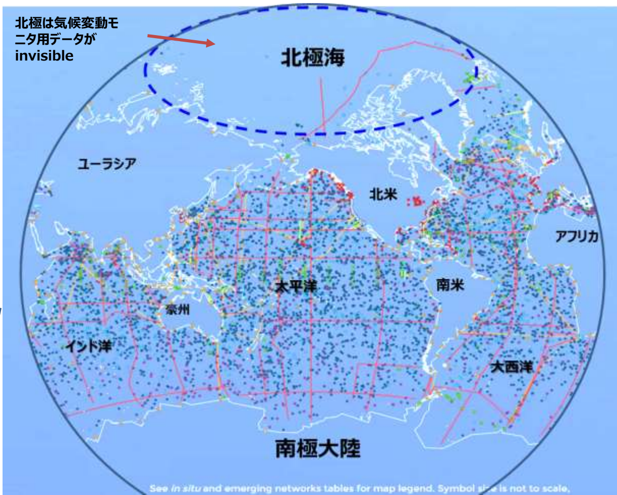
係留観測
