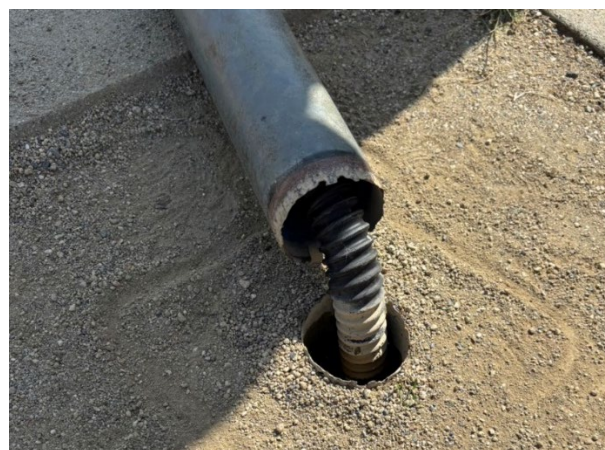
腐食により破損した箇所（支柱の根本）
