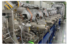
IFMIF/EVEDA開発試験棟で据付調整が進む超伝導高周波加速器
