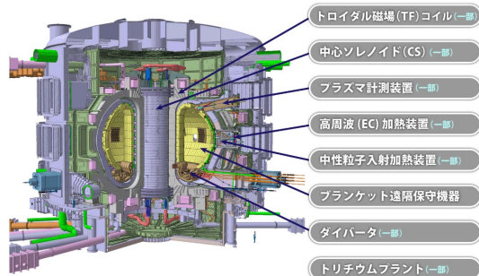
ITERにおける日本の調達機器 ( https://www.fusion.qst.go.jp/ITER/jada/page2_3.html )
