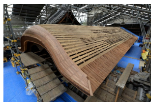
檣皮葺の様子 【重要文化財・妙心寺（京都府京都市）】
