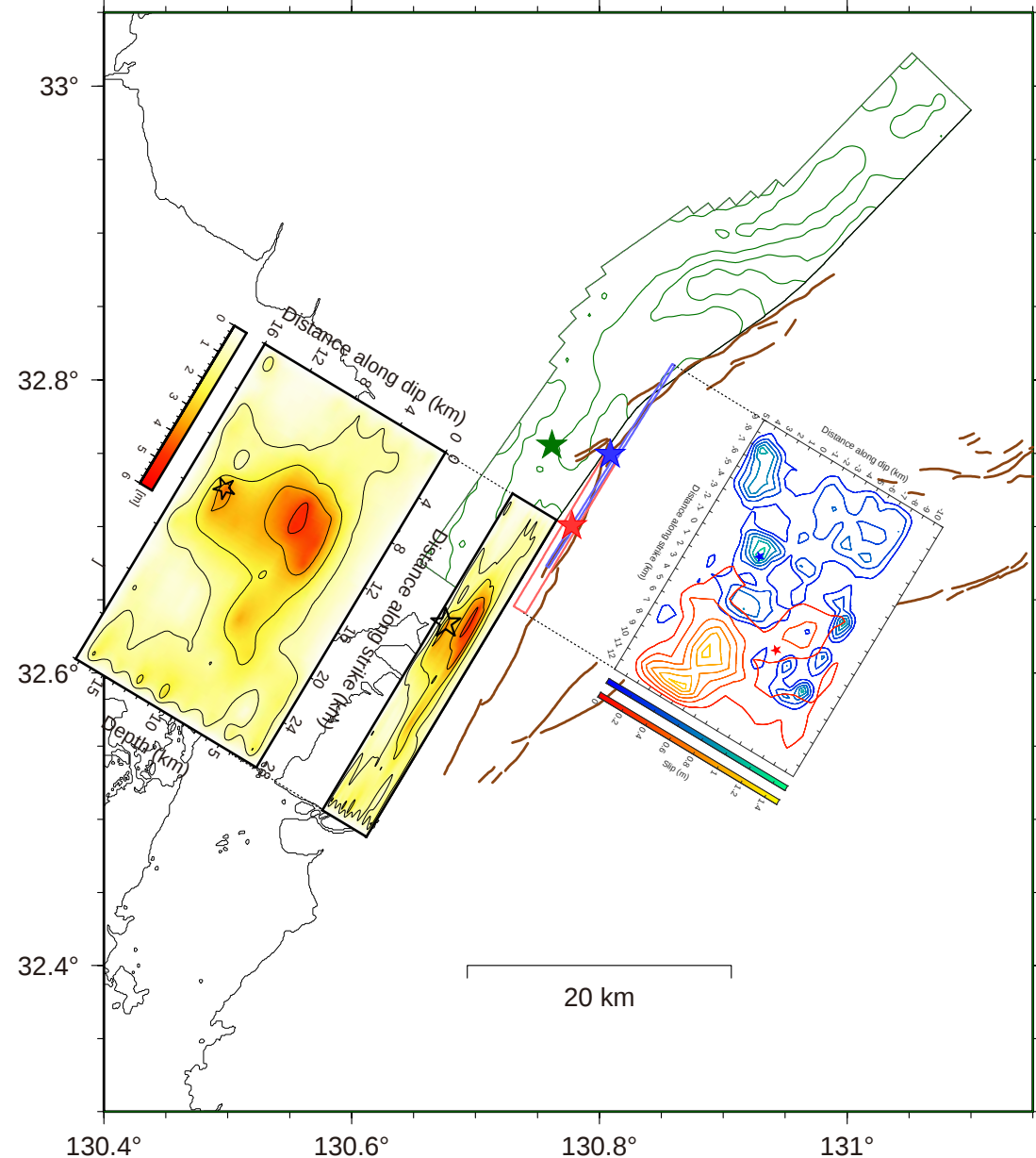
図6：令和8年熊本地震のすべり分布と過去の大規模地震のすべり分布の空間比較。令和8年熊本地震のすべり分布の地表投影をカラーで、破壊開始点を黒星で示す。黒のコンターは1.2m毎のすべり量を示す。2016年4月16日1時25分頃に発生したM j 7.3の平成28年熊本地震の震央を緑の星で、すべり分布を緑のコンターで示す(Kubo et al., 2016, EPS)。緑のコンターは0.8m毎のすべり量を表す。青の星と矩形は2016年4月14日21時26分頃に発生したM j 6.5の地震の震央と断層面を表す。赤の星と矩形は2016年4月15日0時3分頃に発生したM j 6.4の地震の震央と断層面を示す。青と赤のコンターはそれぞれM j 6.5の地震とM j 6.4の地震の0.2m毎の断層すべり分布を表す(Shibata and Aso, 2025, BSSA, 図11に加筆修正)。紫線はAIST (2007)による活断層の地表トレースを表す。
