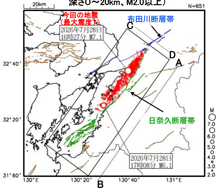
震央分布図
