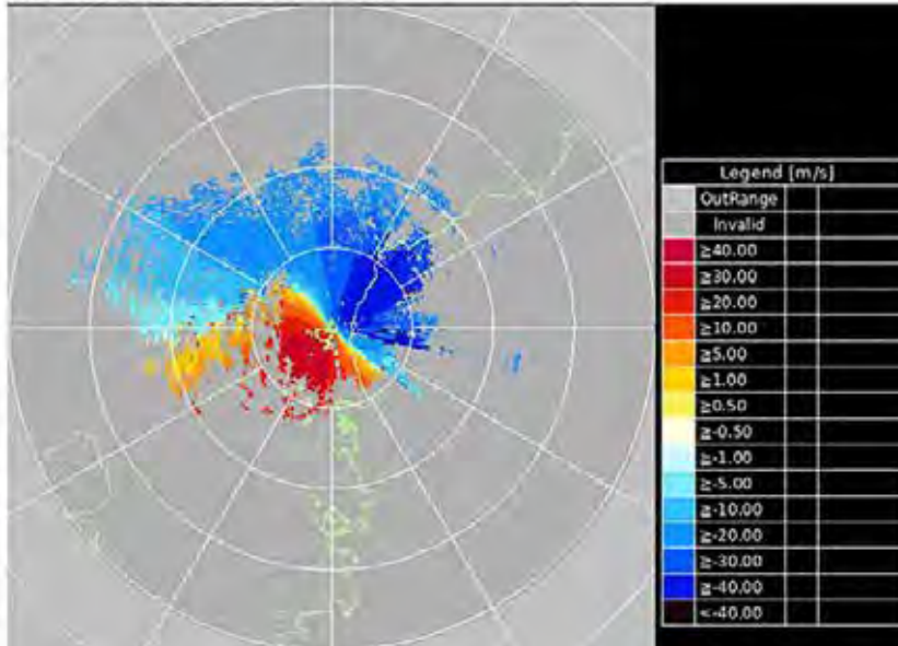
降水粒子のドップラー速度
