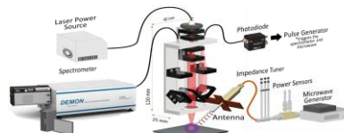
マイクロ波重畳マイクロチップレーザーLIBS実験系 (LIBSプローブはJAEA供給 図：i-Lab社より)
