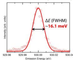
図3 NanoTerasu BL02U 2D-RIXS分光装置のエネルギー分解能 出典：QSTプレスリリースより
