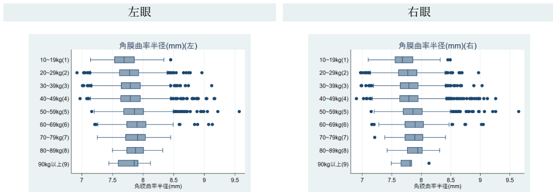
図 6-2-10. 体格（体重）別の角膜曲率半径の分布（箱ひげ図）
