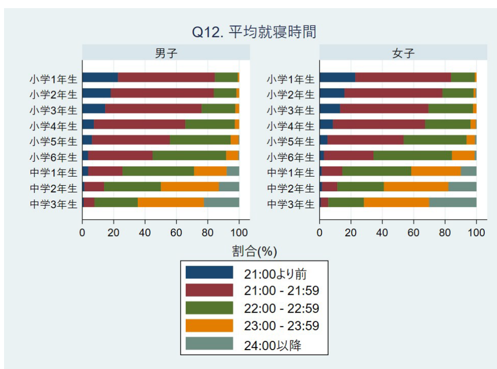
図 5-4-14. アンケート Q12. 「平均就寝時間」 回答の分布
