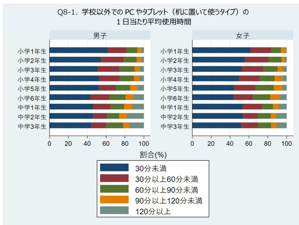
図 5-4-8. アンケート Q8-1. 「学校以外での PC やタブレット（机に置いて使うタイプ）の 1日当たり平均使用時間」回答の分布
