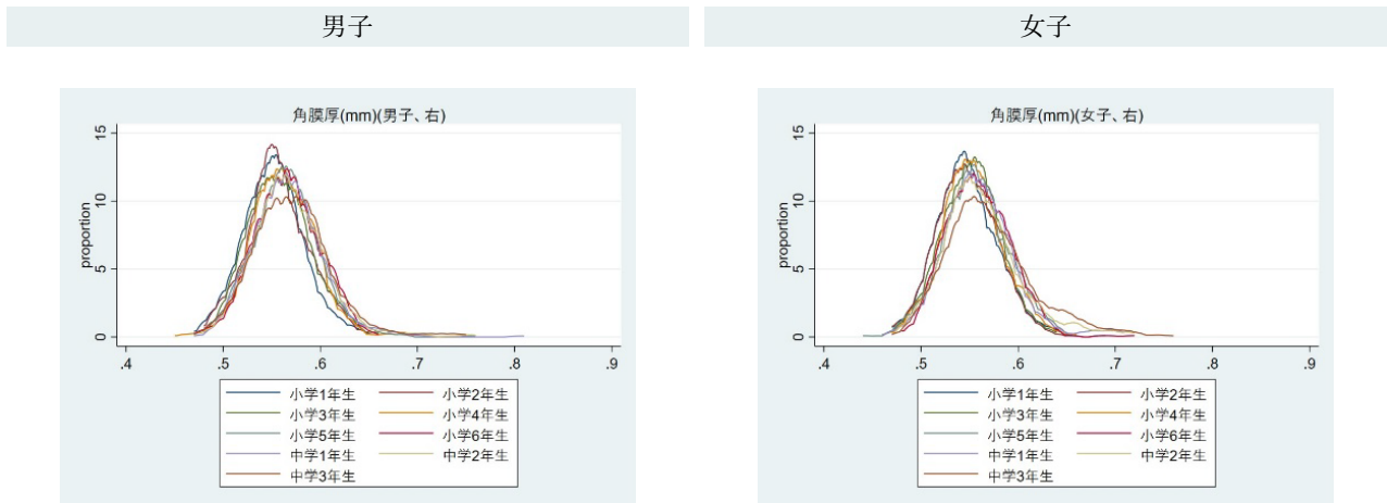
図 5-3-5. 学年・性別の角膜厚 (右) の分布 (カーネル密度関数による表記)
