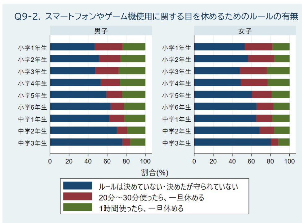
図 5-4-11. アンケート Q9-2. 「スマートフォンやゲーム機使用に関する目を休めるためのルールの有無」 回答の分布
