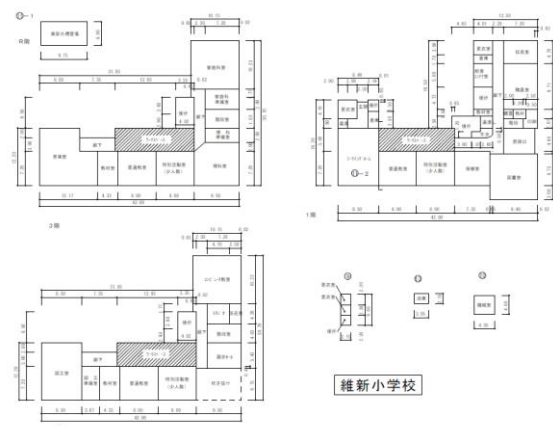
校舎の平面図
