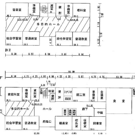
校舎等の平面図
