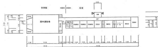
校舎等の平面図
