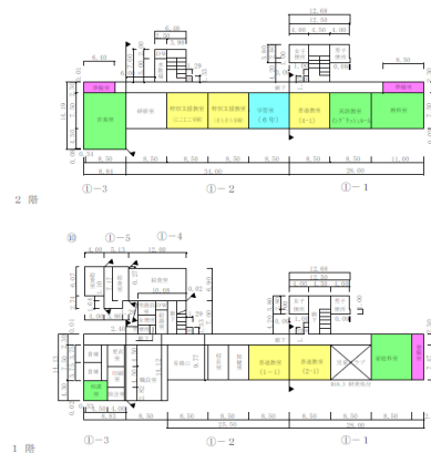
校舎平面図(1階・2階 詳細は上記URLをご確認ください)
