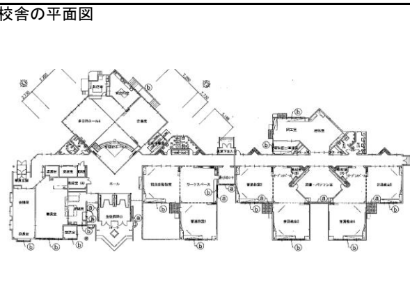
校舎の平面図
