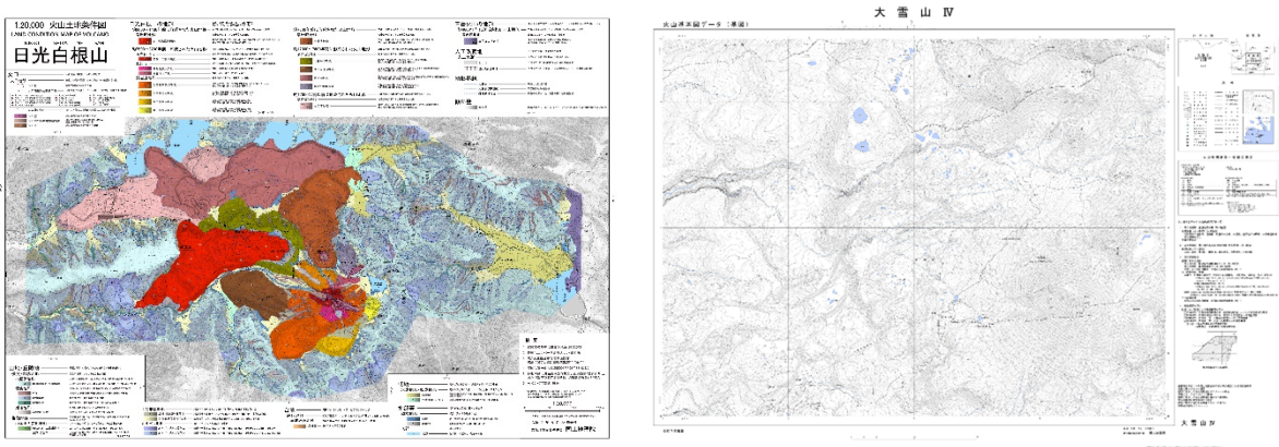
図 3 火山土地条件図「日光白根山」（左）、火山基本図「大雪山Ⅳ」（右）
