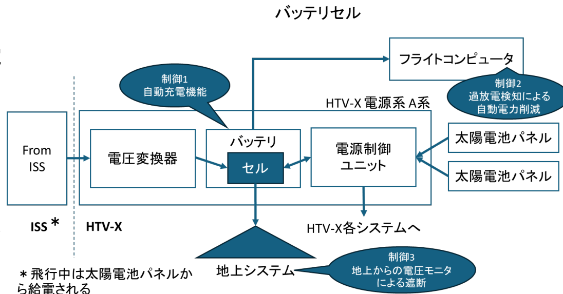
HTV-X電源系 制御図 (過放電防止制御の例)
