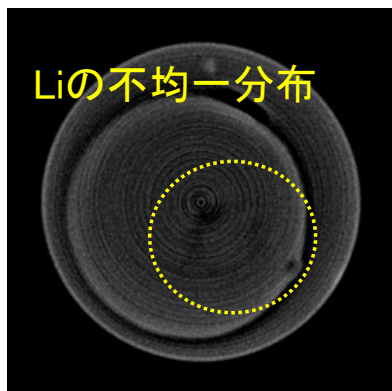
中性子ラミノグラフィ (分解能20 \mu m)
