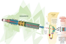
DONES加速器
