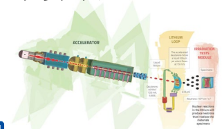
DONES加速器
