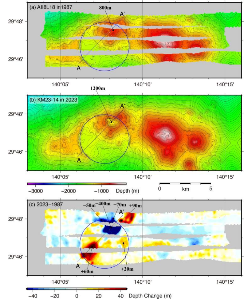
地形変化 (Fujiwara et al., 2024)
