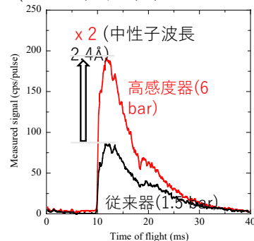
(1x1mm ダイレクトビーム@BL17)
