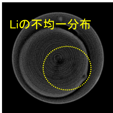
中性子ラミノグラフィ (分解能 20\mu\text{m} )
