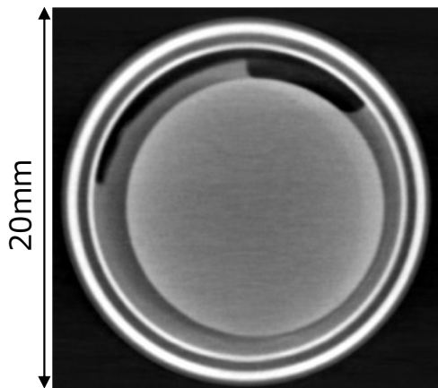
中性子CT
