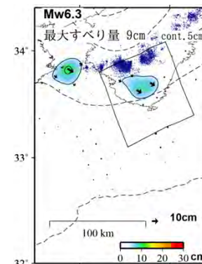
紀伊半島SSEのすべり分布 (2025年1月まで)
