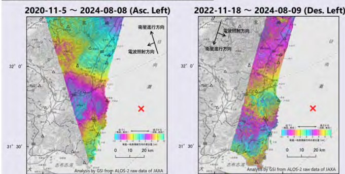
干渉解析結果(2024年8月8日, 8月9日)
