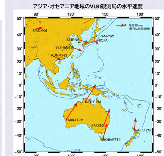
グローバル解析結果
