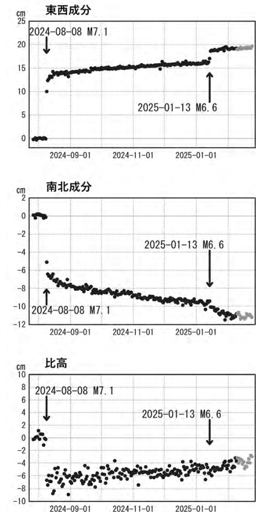
電子基準点「宮崎」における 3成分の時系列変化
