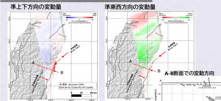
2.5次元解析結果(2024年4月4日, 4月5日)
