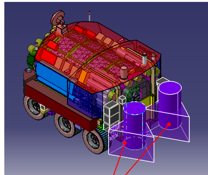
月面展開ペイロード (後面2カ所)
