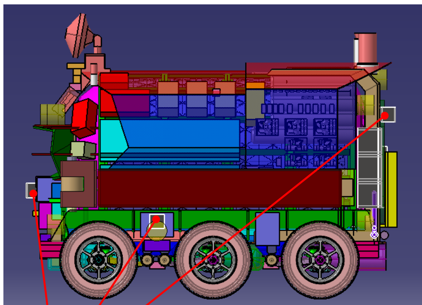
船外ペイロードインタフェース (前後左右面にそれぞれ1カ所、計4カ所)
