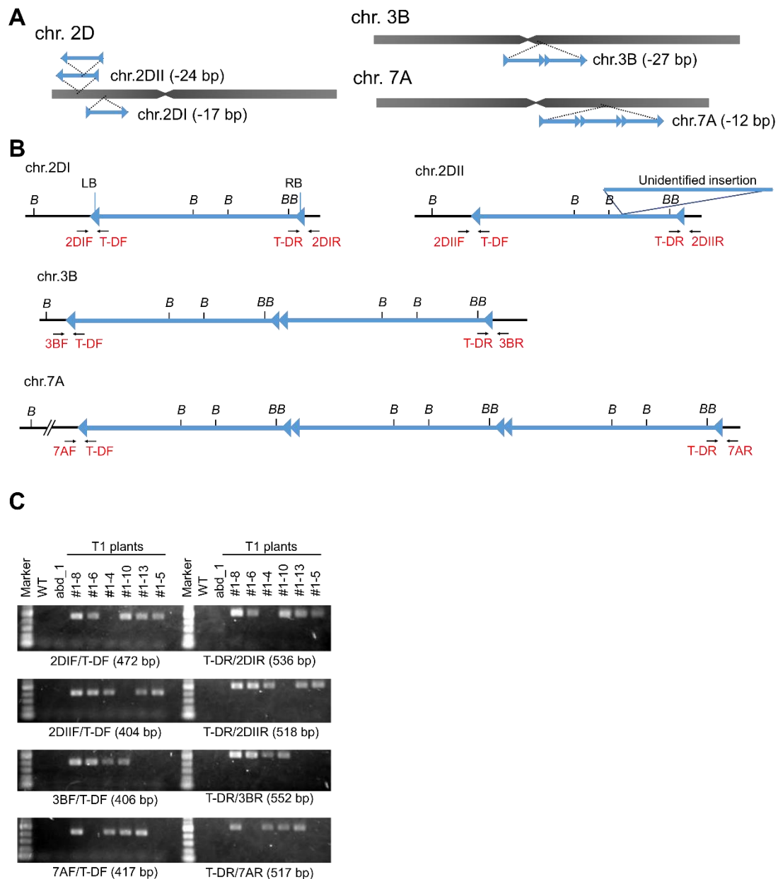
図 7 ゲノム編集システム作成において用いた T-DNA の挿入位置の特定
