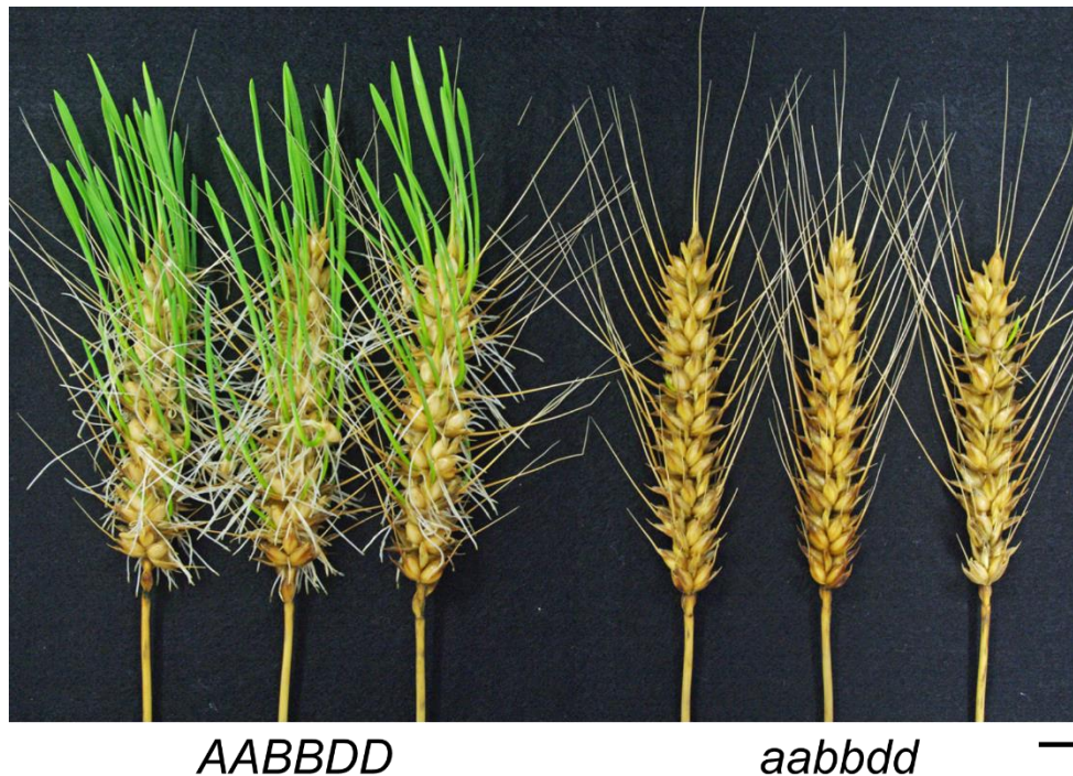
図 11 穂を立てた条件での発芽試験
