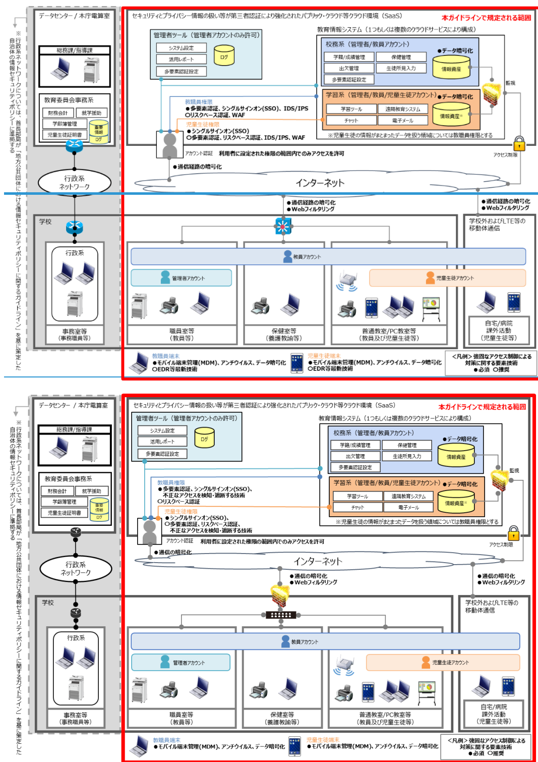
図表 13 強固なアクセス制御による対策を講じたシステム構成例
