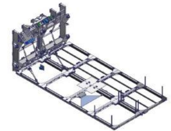
パネル展開状態 (ISS離脱後)
