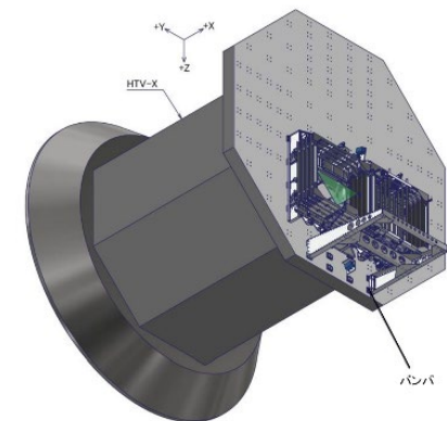
HTV-XのDELIGHT搭載位置
