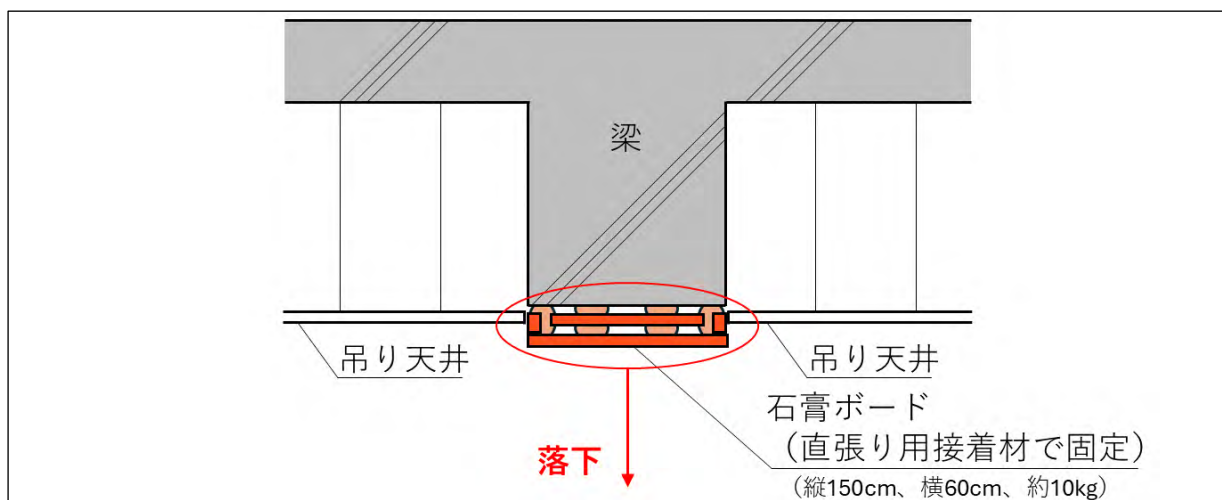
天井ボード落下箇所（概略断面図）
