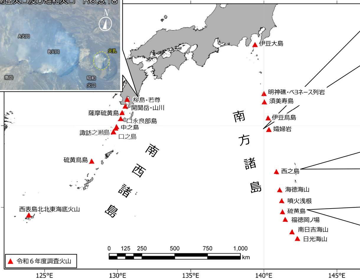
桜島の南岳火口及び昭和火口 R6.3.18
