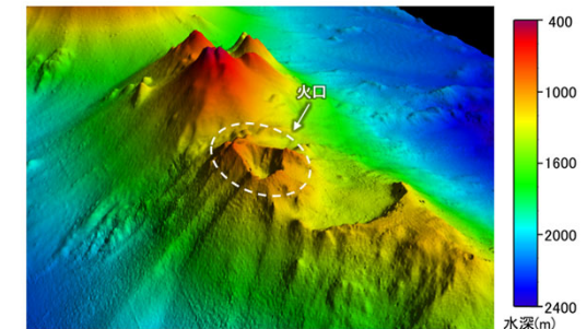
鳥島近海（壱婦海山）の海底地形
