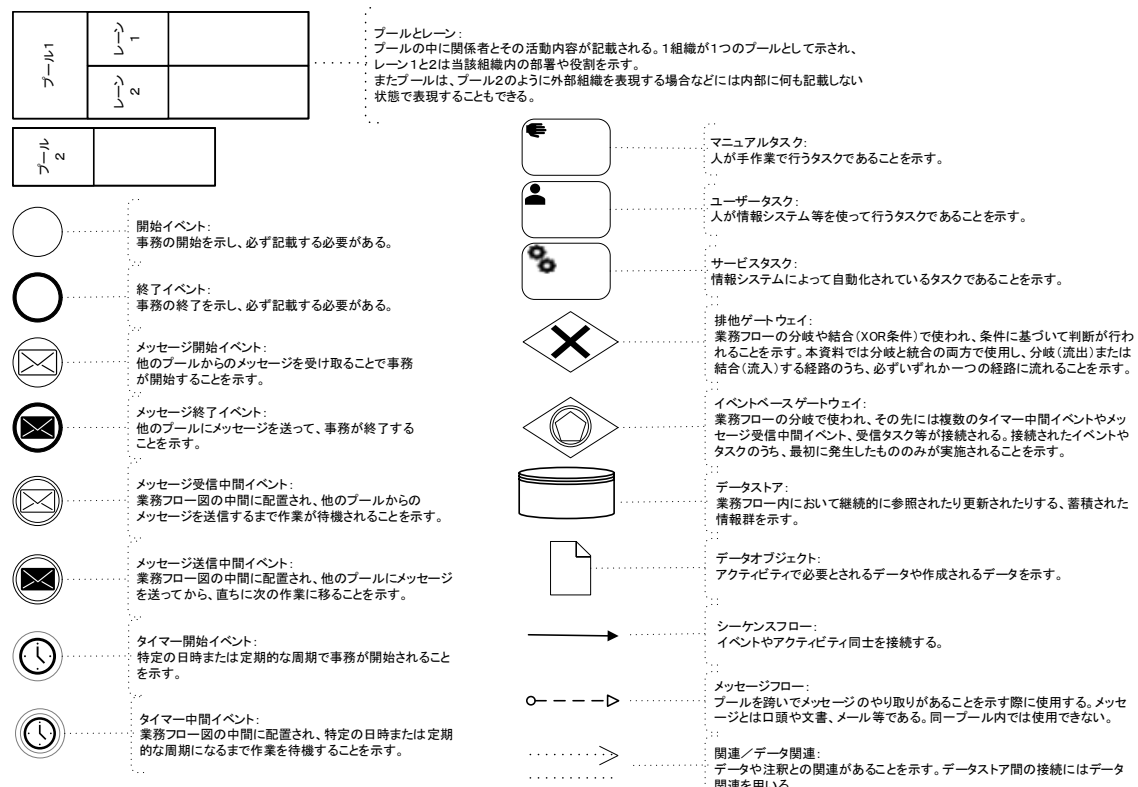
BPMN 凡例
