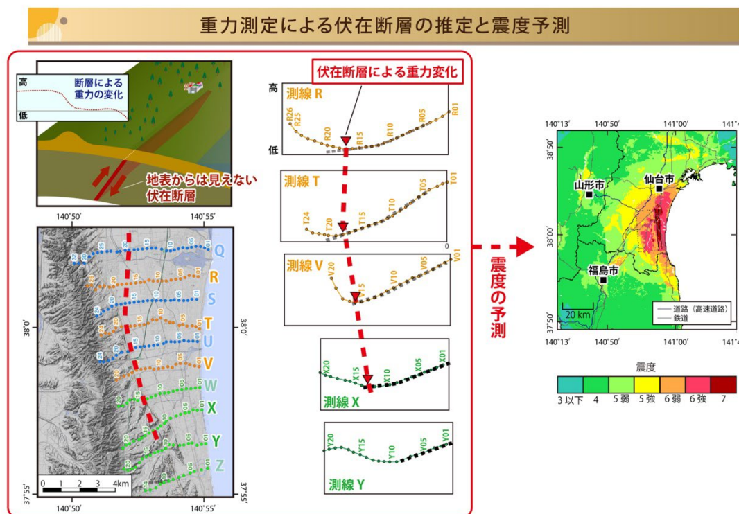
図4-8 重力測定による伏在断層の推定と震度予測。仙台平野南部において，反射法地震探査で確認されている伏在活断層に伴った重力変化を追跡した結果，伏在活断層による重力変
