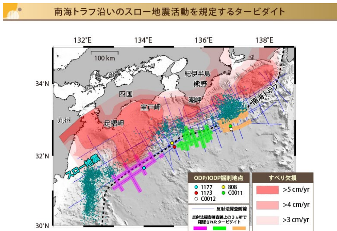
図 4-7 南海トラフ沿いのスロー地震活動を規定するタービダイト。南海トラフに沿って沈み込む深海堆積物を調査した結果、砂層に富むタービダイト（反射法探査測線上の桃、緑、橙色の領域）が、スロー地震活動の静穏域（水色の丸がない領域）、すなわちプレート間固着の強い領域（赤のグラデーションが濃い領域）に集中して分布することを発見した。透水性の優れたタービダイトがプレート境界断層の間隙水圧を低下させることで、断層面のせん断強度が大きくなり、スロー地震活動が静穏化した可能性を示唆する。
