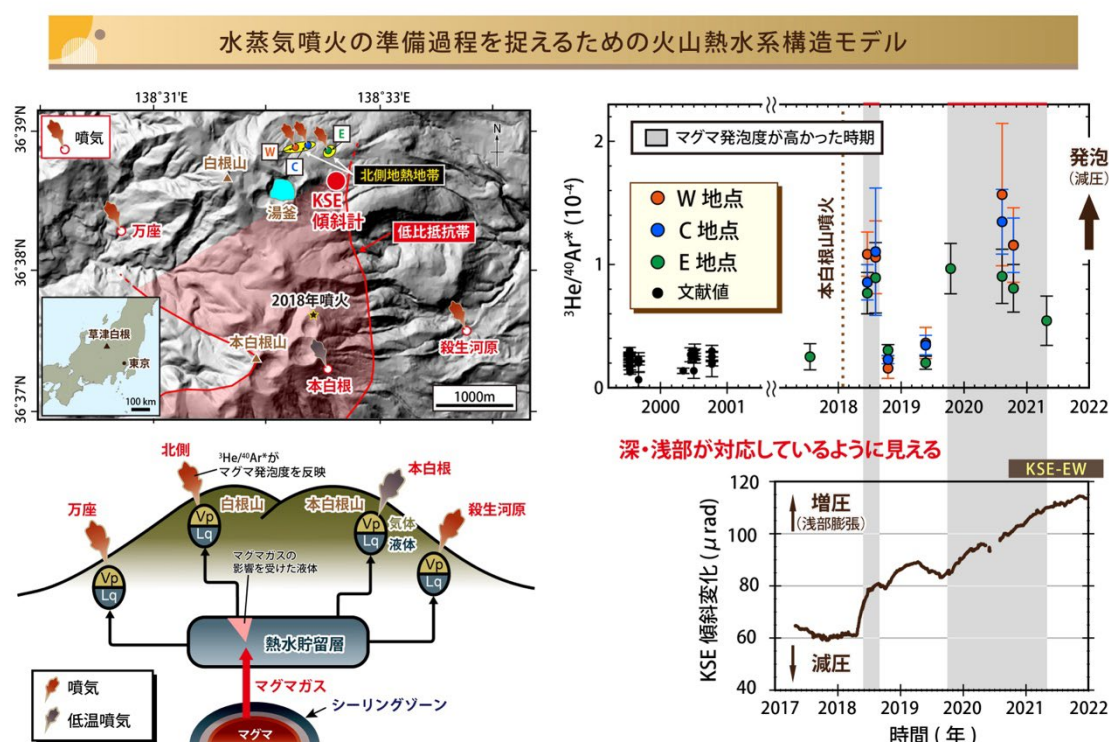
図2-2. 水蒸気噴火*の準備過程*を捉えるための火山熱水系構造モデル。草津白根山の湯釜火口北側の噴気について、 ^3\text{He}/^{40}\text{Ar} 比に基づきマグマ発泡度の変化が検出された。発泡度変化のタイミングは浅部熱水だまりの膨張・収縮とよく一致しており、同火山の活動の活発化を駆動するマグマ～浅部活動の物質科学的*なつながりが確認できた。 ^3\text{He}/^{40}\text{Ar} 比 ( ^{40}\text{Ar}^* はマグマ由来の ^{40}\text{Ar} を意味する) というこれまで使われていなかった指標が火山活動活発化と関係していること、さらにマグマの発泡で説明できることを示した。草津白根山のような熱水が卓越している火山の活動活発化にマグマ (おそらく熱水系より深部) の寄与を示唆した意義もある。希ガスなので複雑な反応を考える必要がなく、今後、火山活動モニタリングの指標の一つとして活用が期待できる。
