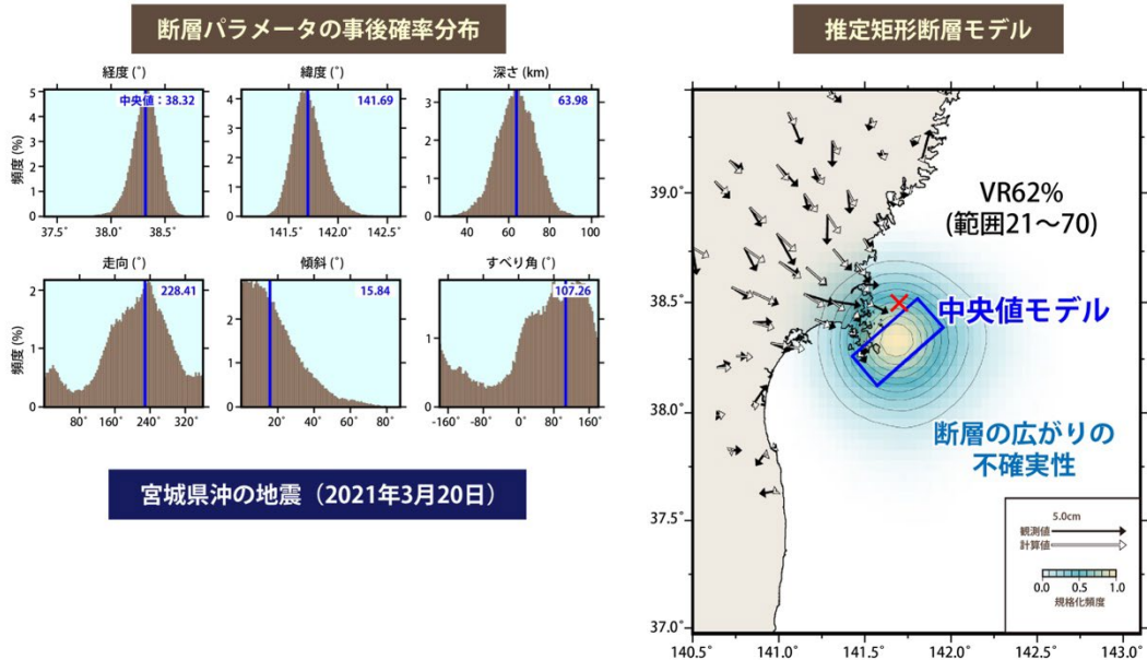
図 2-7 高速な断層推定。REGARD による 2021 年 3 月 20 日に発生した宮城沖地震の地殻変動から断層パラメータを推定したもの。左は断層パラメータの事後確率分布、右は推定された矩形断層モデルの位置とその広がりの不確実性を示す。左の青線は中央値で、右上にその数値を示す。東北大学で開発された推定パラメータの不確実性を評価できるプログラムを国土地理院に技術移転した。従来法からの置き換えに向け、試験運用中である。
