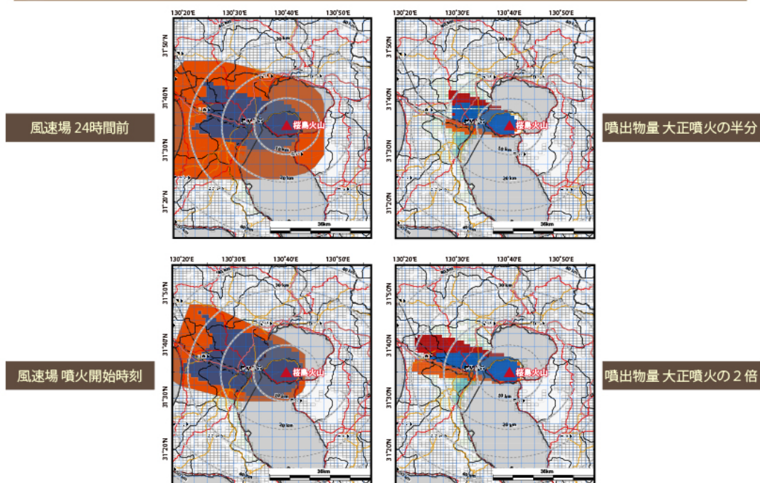
図 4-11 降灰予測シミュレーションにおける風速場・噴出物量の重要性。鹿児島市街地に影響が及ぶ風速場（2018 年 7 月 15 日）において桜島南岳山頂火口において大規模噴火が発生した場合における降灰危険度予測（右上，右下）。降灰危険度予測を基に避難すべき範囲の余長の持たせ方の変化（左上，左下）。噴火の 24 時間前予測では余長域が広いが，現時点予測では余長域が狭くなるように設定されている（左図の赤色の範囲）。
