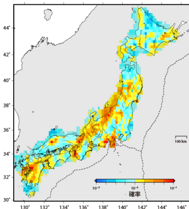
図 4-6 測地データと地震活動度から求めた内陸域での地震発生確率。GNSS データと背景地震活動データから、 M_{JMA}6.0 以上の地殻内地震の 30 年発生確率を色で示す。赤い色の地域ほど、発生確率が高い。平均変位速度*が速い活断層では、余震の継続時間が短い傾向が見られた [DPRI05] 。
