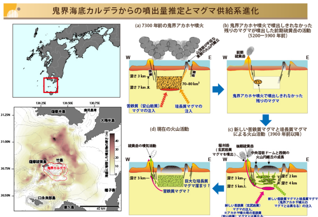
図 4-3 鬼界海底カルデラからの噴出量推定とマグマ供給系進化。反射法地震探査により得られた層構造と噴出物との対比から、2 回の大規模火砕流噴火に相当する堆積物が海底に厚く堆積しており、噴出量は 71 km³ 以上であると推定された。噴出物の分析からは、(1)
