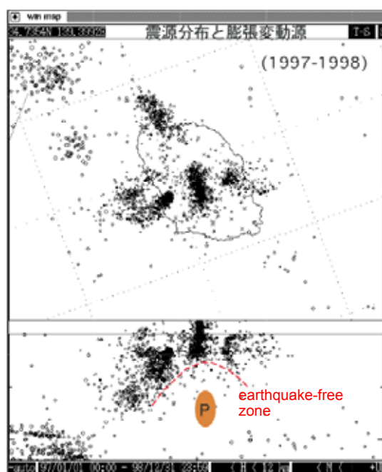
図32 伊豆大島周辺の震源分布。Pは推定された山体膨張源の深さ範囲
