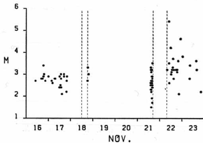
図 16 1986 年噴火時の M—T ダイアグラム (沢田・他、1988)
