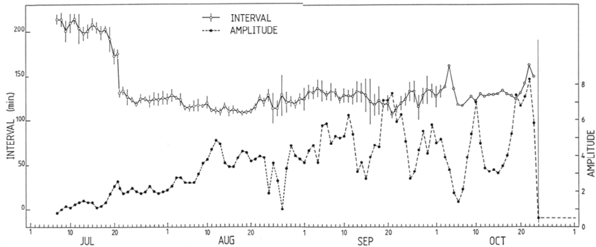
図9 1986 年山頂噴火に前駆した微動の振幅と発生間隔の日平均値 (渡辺、1987)
