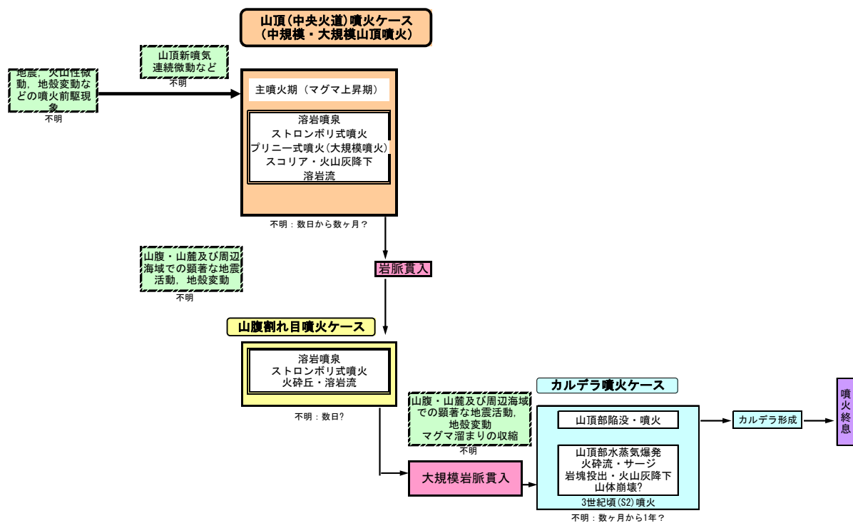
図3 S2（約 1700 年前）噴火の推移
