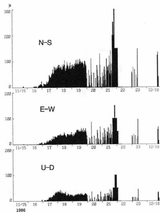
図 20 1986 年噴火時の火山性微動の振幅変化（山里・他、1988） 傾斜変動（図 6）と同期して連続微動が間欠的になった
