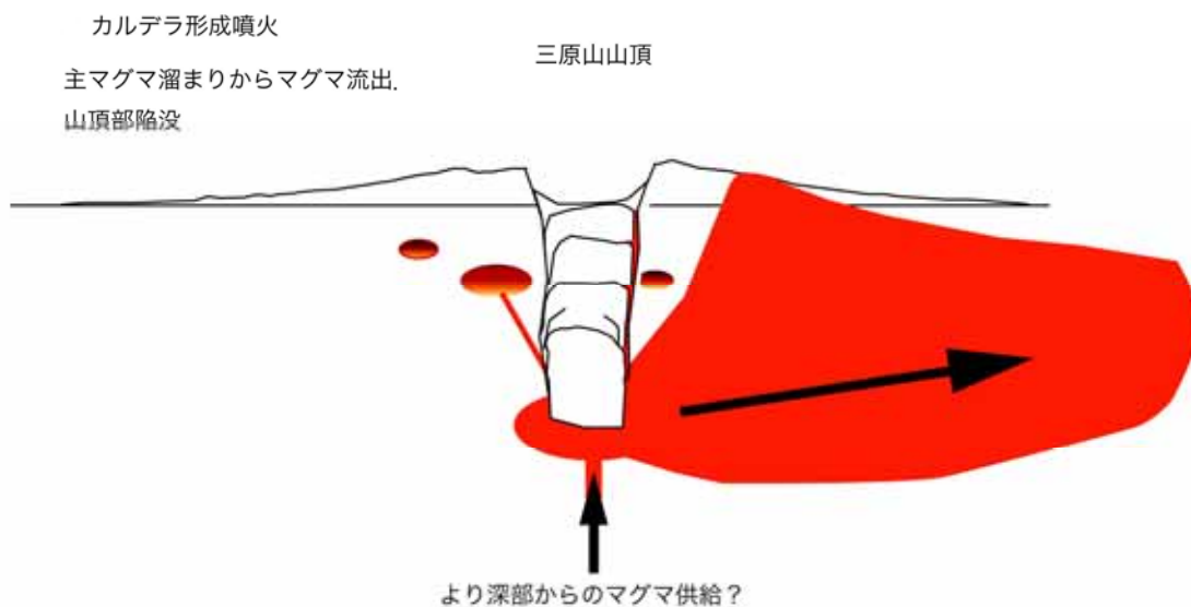
図 31 カルデラ噴火のマグマ供給・排出系モデル (川邊 原図)
