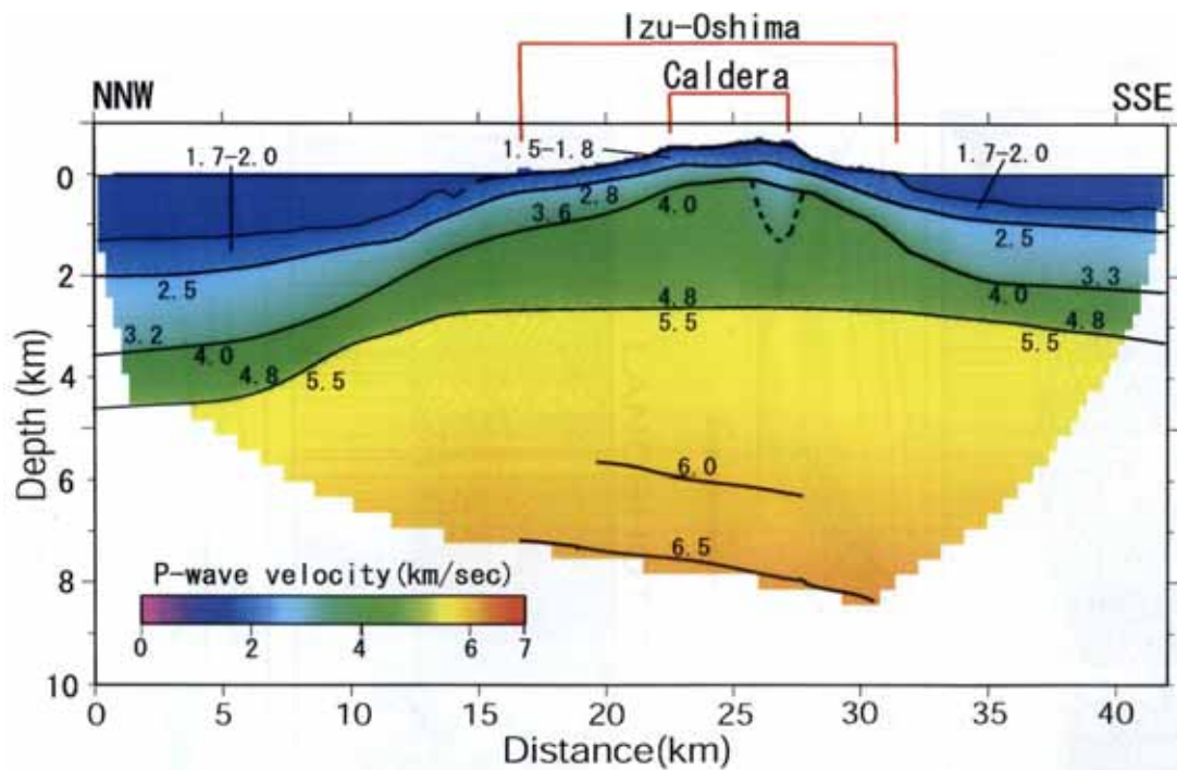
Fig5-27 本研究で求めたP波速度構造 図中の数値はP波速度(km/s)である。第2層、第3層上面はカルデラ下へ向けて盛り上がっている。 第4層上面は伊豆大島島内下では水平になっている。第3層上面の点線で表示している部分は低速度領域である。 深さ6.0km付近と深さ8.0km付近に反射面がある。
