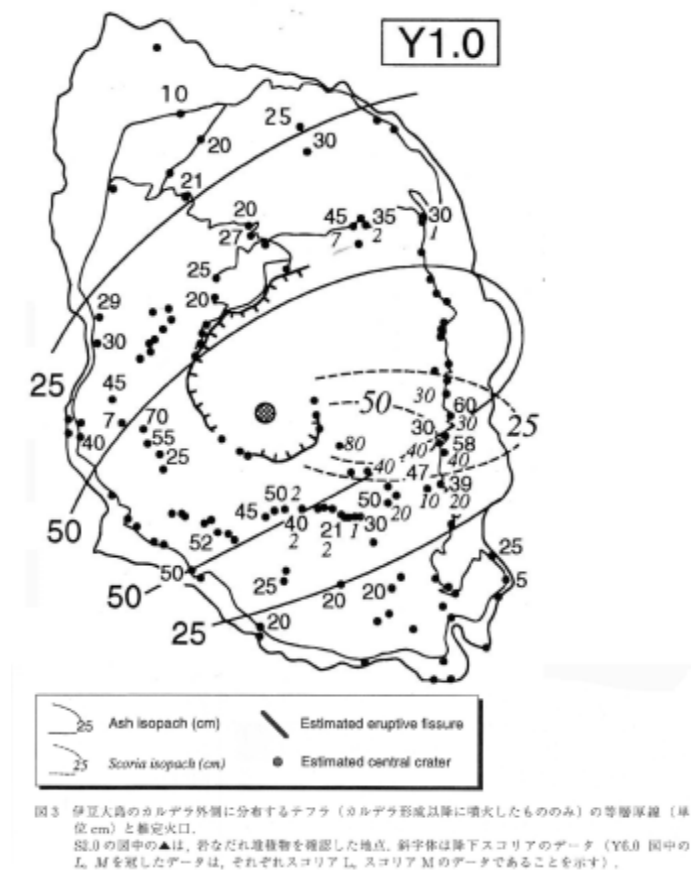
図11 Y 1 基底スコリア(破線)および火山灰(実線)の層厚(cm)(小山・早川、1996)
