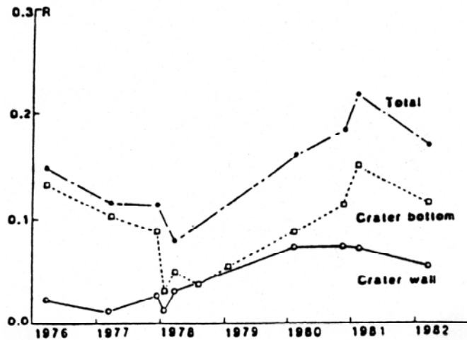
図6 1986年噴火前の三原山頂火口底における熱異常域の変化(鍵山・辻、1987)
