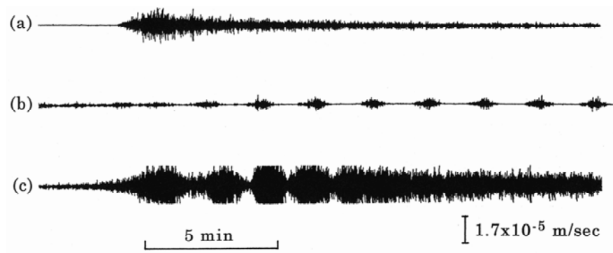
図10 1986年噴火前に発生した微動のカルデラ内における観測波形の推移（渡辺、1998）
