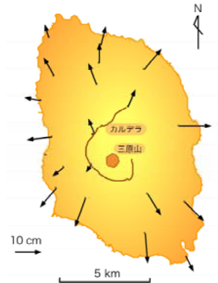
図 34 1988 年～1994 年の期間の水平変位ベクトル。 膨張変動源は、カルデラ北部の深さ 6～8 km と推定される（国土地理院、1996）
