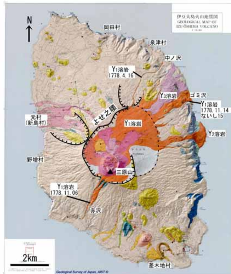
図12 伊豆大島火山地質図(川辺、1998). Y 1 溶岩の流下の日付、当時の地名ほかを加筆
