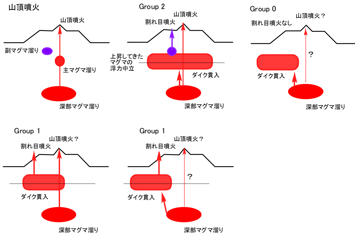
図 17 割れ目噴火様式の模式図
