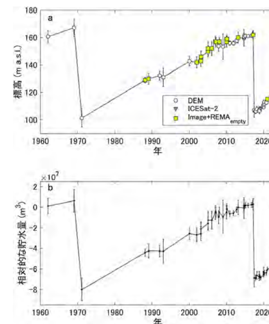
図2：1962～2021年の (a) 湖面標高及び (b) 貯水量。50年かけて貯まった湖水が突発的に放出された様子が見て取れる。
