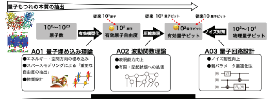
図2 本領域で構築する第一原理計算の新しい学理
