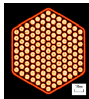
燃料集合体 X線CT画像
