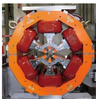
六極電磁石 各 10 \times 16 = 160 台
