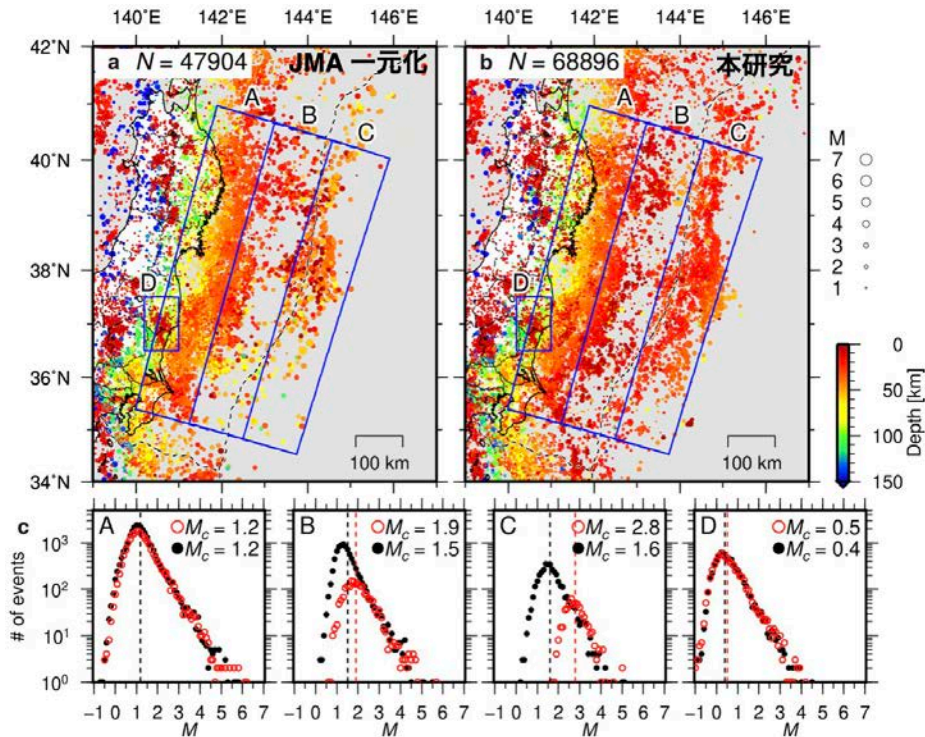
図22. S-netを含む基盤的地震観測網のデータから、機械学習による自動ノイズ除去法を適用して作成した震源カタログ (Tamaribuchi et al., 2021より改変、気象庁 [課題番号: JMA_01] )
