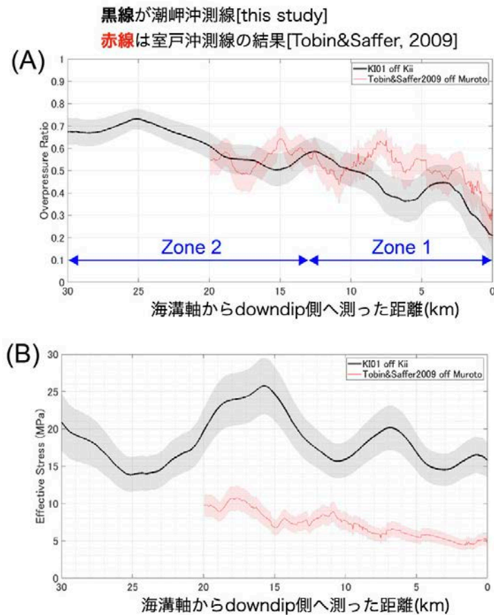
図11. P波速度構造から推定した潮岬沖の(A)過剰間隙水圧比と鉛直有効応力 (Yu et al., 2021より改変、東京大学地震研究所 [課題番号：ERI_12] ) Zone1とZone2の区分はデコルマの物性や付加体の層厚変化に基づく。
