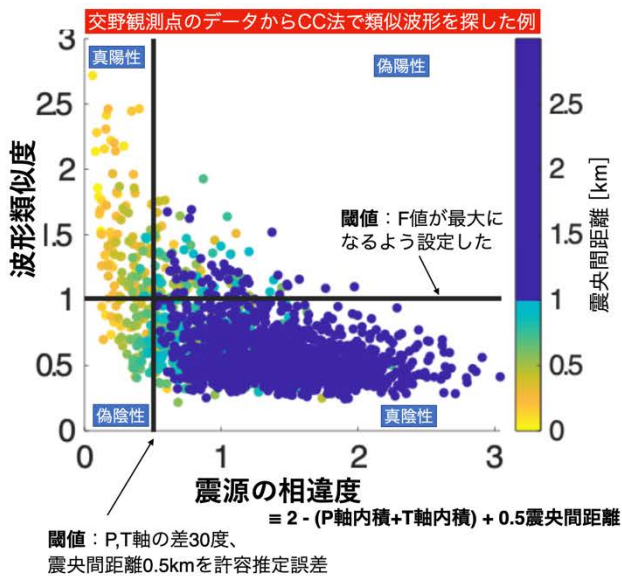
図21. 波形類似度と震源の相違度の比較（高山・他，2021より改変、立命館大学 [課題番号：RTM_02]）
