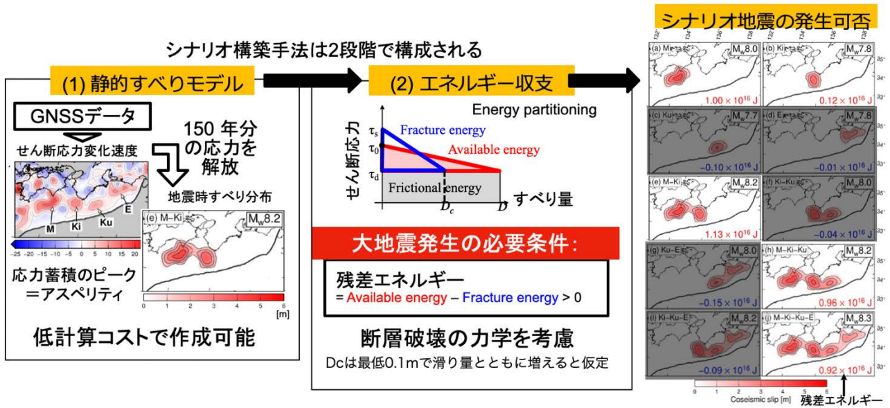
図14. 滑り遅れレートに基づいてエネルギー収支を考慮した地震発生シナリオの評価法 (Noda et al., 2021より改変、気象庁 [課題番号: JMA_01])
