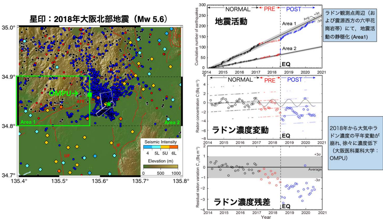
図31. 2018年大阪府北部地震に先行した大気中ラドン濃度変動 (Muto et al., 2021より改変、東北大学 [課題番号: THK_10])
