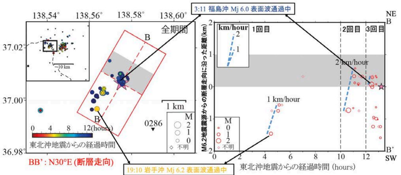
図19. 2011年M9東北沖地震の13時間後におきた長野県北部M6.2地震の前震活動 (Shimojo et al, 2021より改変、東京大学地震研究所 [課題番号：ERI_13])
