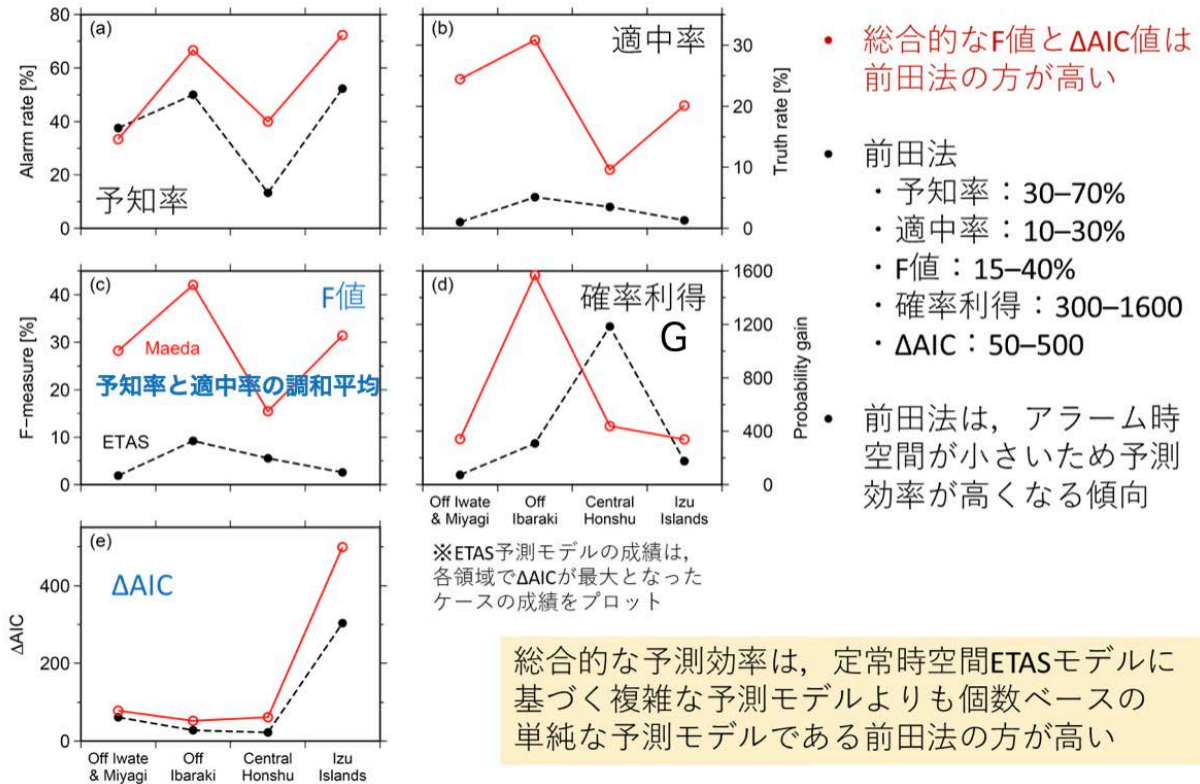
図18. 岩手・宮城沖、茨城沖、本州中部、伊豆諸島での前田法とETASモデルによる短期地震予測の成績 (Hirose et al, 2021cより改変、気象庁 [課題番号：JMA_01]、東京大学地震研究所 [課題番号：ERI_13])
