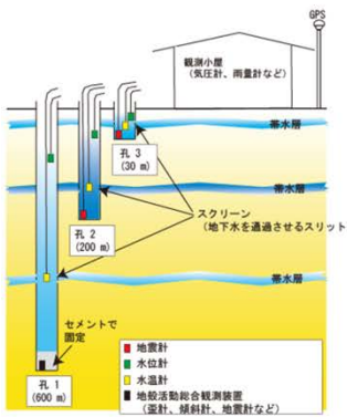
産総研の地下水・ひずみ総合観測施設
