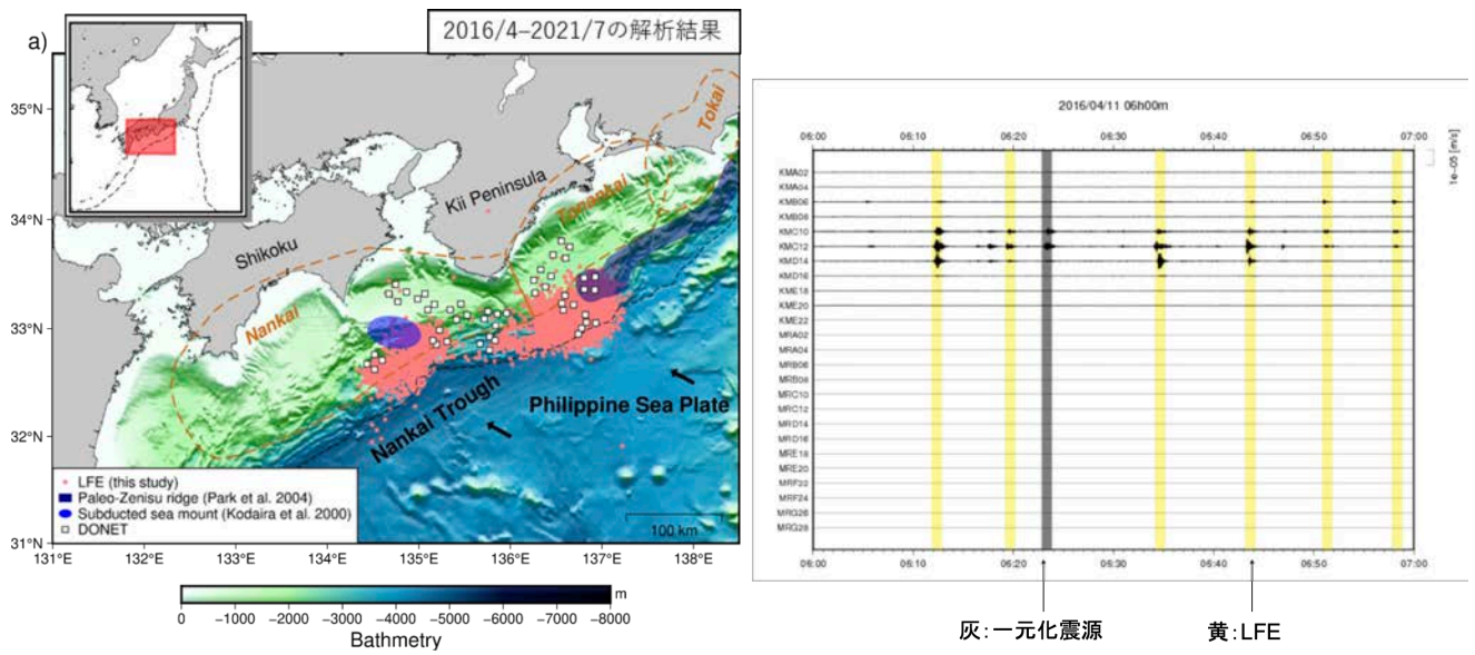
図 8. 最大振幅とエンベロップ相関を用いたハイブリッド法を用いて検出された浅部LFE（溜瀨・小木曾，2021bより改変、気象庁〔課題番号：JMA_01〕） ピンク点は本手法により検出された浅部低周波地震。薄い青色はそれぞれ沈み込んだ海山や海嶺、四角印はDONETの観測点を表す。
