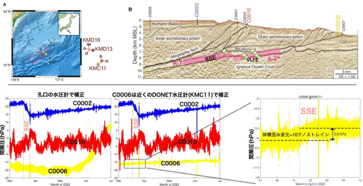
図 7. 間隙水圧変化で捉えた浅部SSE (Ariyoshi et al., 2021より改変、東北大学理学研究科 [課題番号: THK_09])
