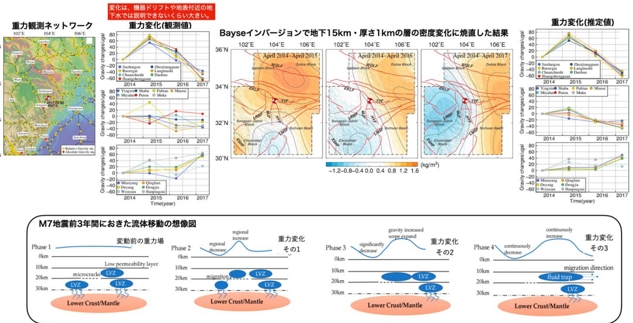
図29. 2018年8月8日チベット高原東縁Jiuzaigou地震(M7)数年前の広域重力変化 (Yang et al., 2021より改変、東京大学地震研究所 [課題番号: ERI_13] )
