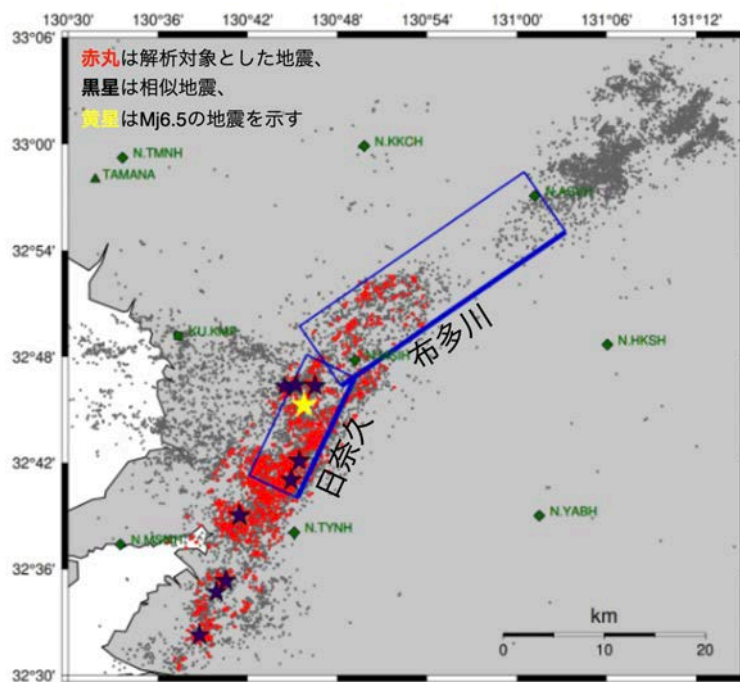
図2. 2016年熊本地震震源域周辺で発生した相似地震の探索 (森・平松, 2021より改変, 東北大学理学研究科 [課題番号: THK_09])
