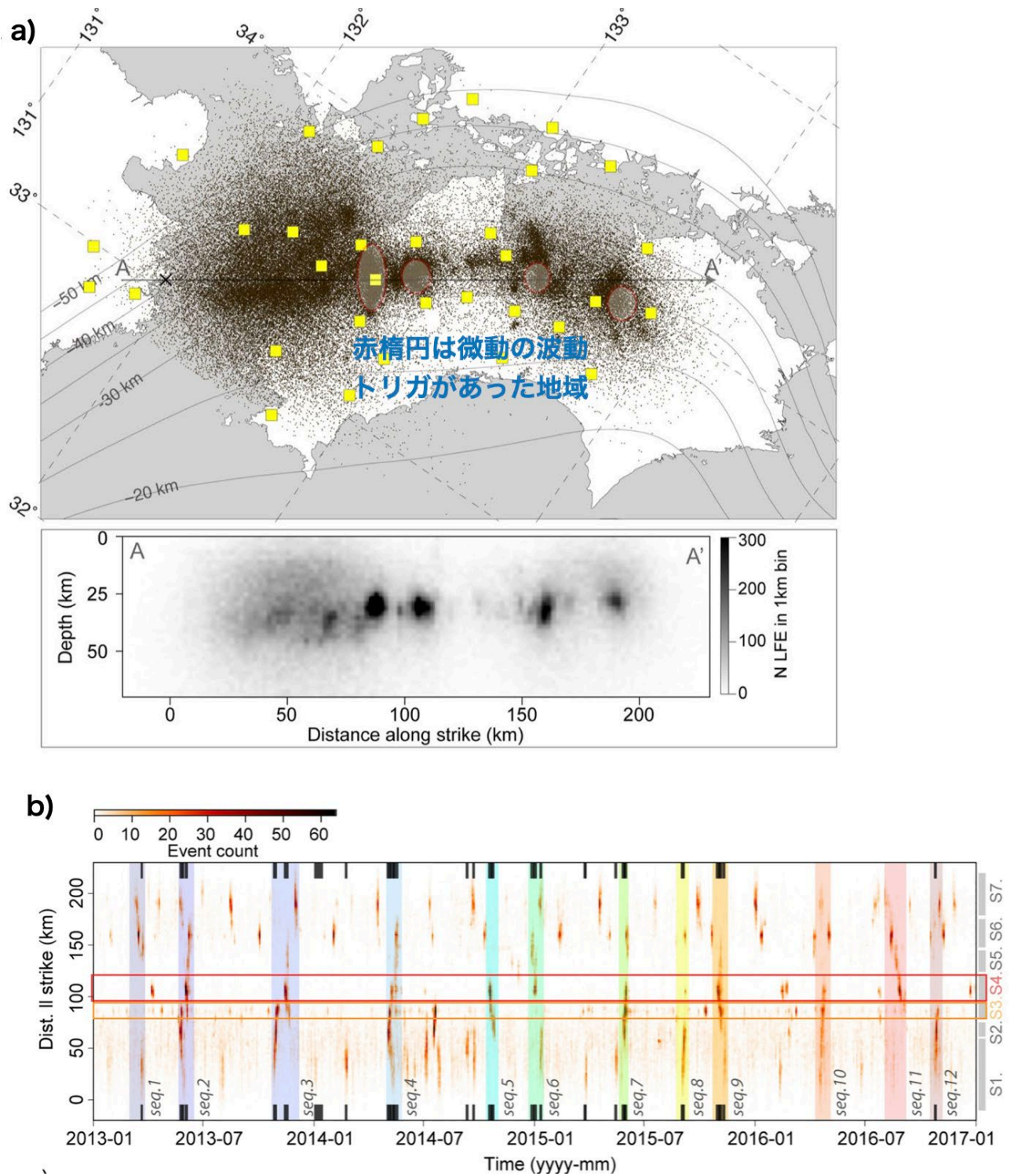
図 5. テンプレートを使わない新手法で検出された四国地域のLFE (Poiatea et al., 2021より 改変, 東京大学地震研究所 [課題番号: ERI_12])
