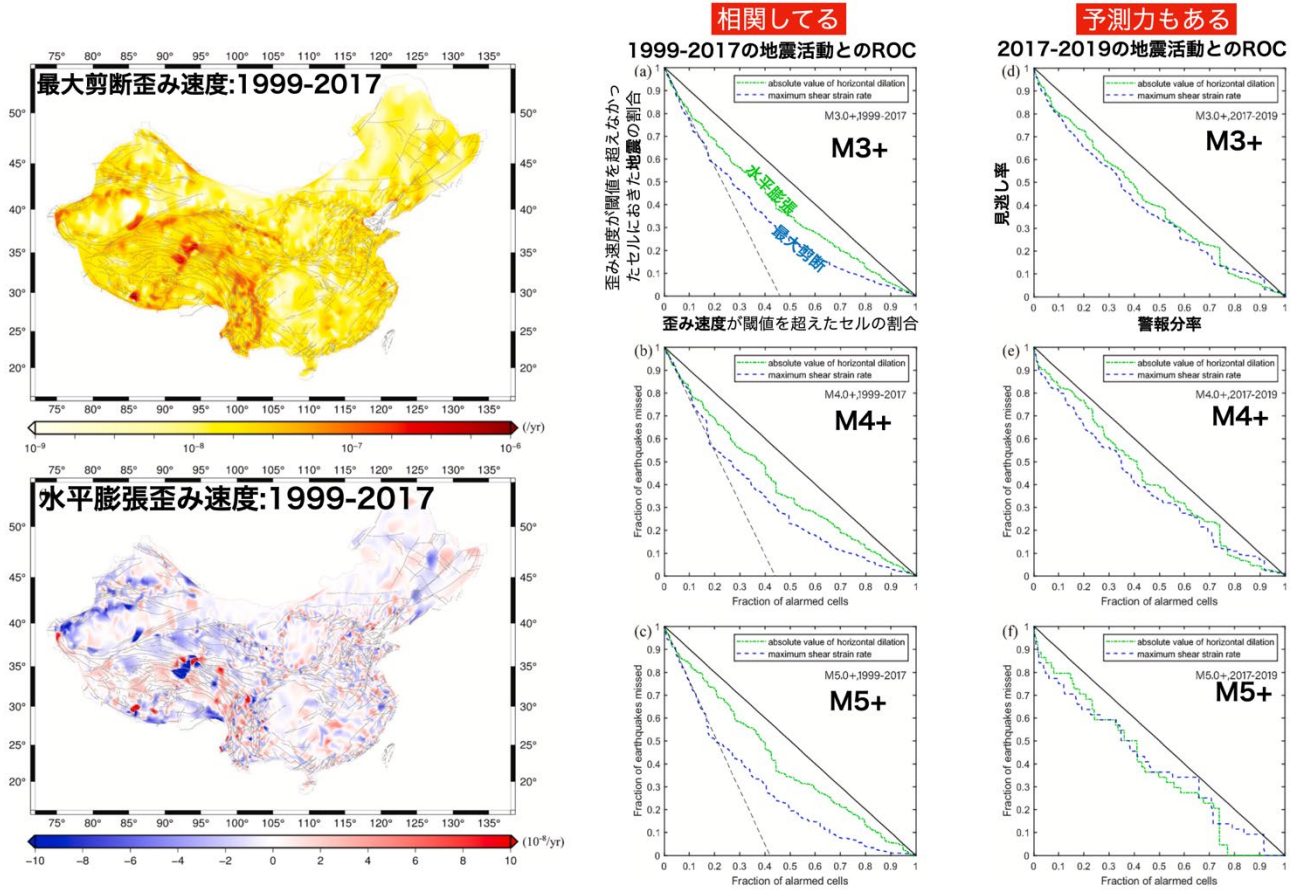
図30. 中国全土のGNSS歪みレートと背景地震活動の比較 (Xiong et al., 2021より改変、東京大学地震研究所 [課題番号: ERI_13])
