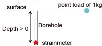
図33. 設置深度を考慮した海洋潮汐による理論ひずみの計算（Kamigaichi et al., 2021より改変、産業技術総合研究所 [課題番号：AIST09]）
