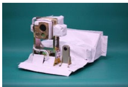
SOLISSフライトモデル
