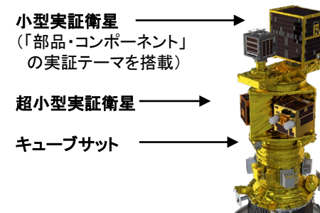
革新的衛星技術実証3号機の搭載イメージ
