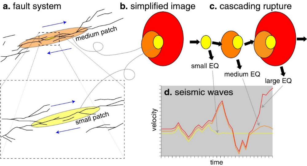
推測される破壊成長のイメージ
