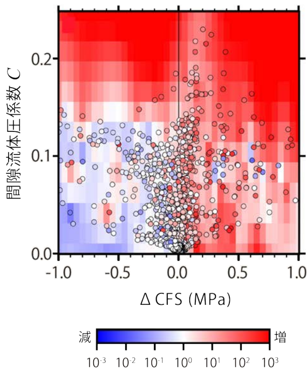
地震活動度の変化と \Delta CFS 及び地震前の間隙流体圧の関係
