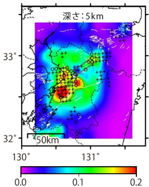
地震前の間隙流体圧力場と地震活動度の変化
