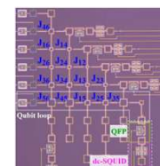
超伝導量子アニーリングマシンチップ
