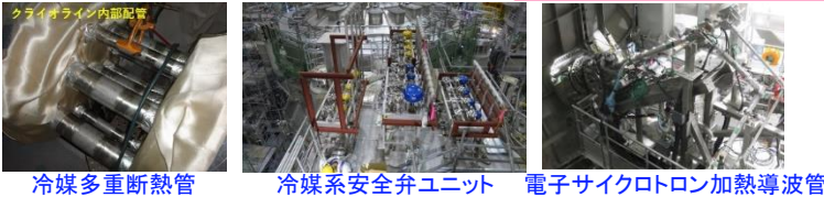
クライオライン内部配管 冷媒多重断熱管 冷媒系安全弁ユニット 電子サイクロトロン加熱導波管
