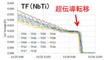
超伝導コイルの冷却による転移の確認
