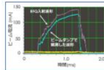
実験データの例 (RFQ前後でのビーム電流波形)
