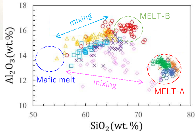
宝永噴火の斑レイ岩捕獲岩
