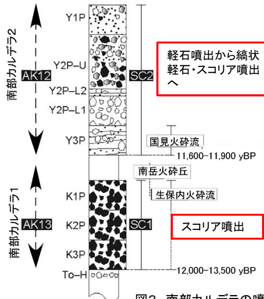
図3. 南部カルデラの噴火推移と本質物の時間変化
