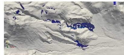
1991年6月3日火砕流堆積物分布
