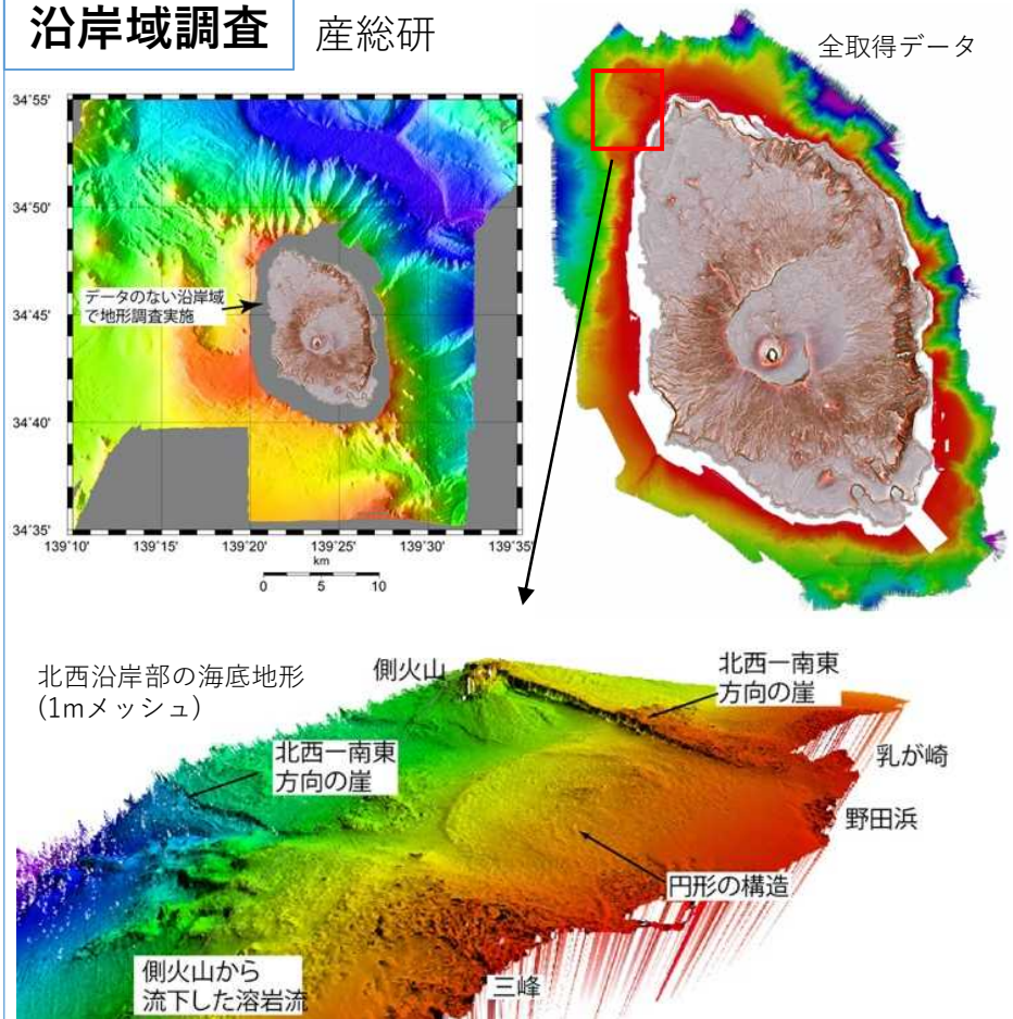
伊豆大島：沿岸海底部の活動度調査
