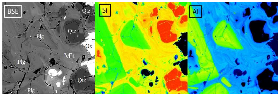
石英を含むクリスタルマッシュ試料 (FjGB18) のBSE像と元素濃度マップ
