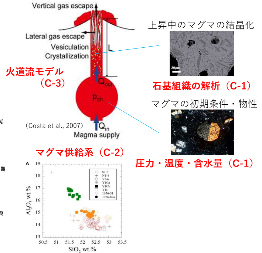
噴火活動履歴（C-2）
