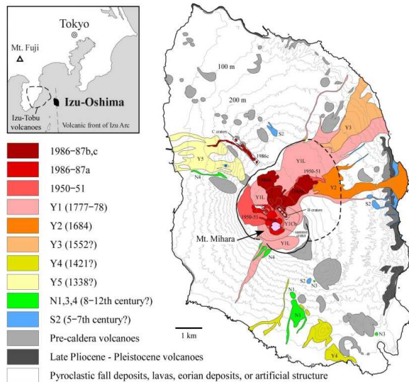
火山地質図（川辺，1998）
