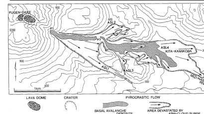
1991年6月3日火砕流堆積物分布
