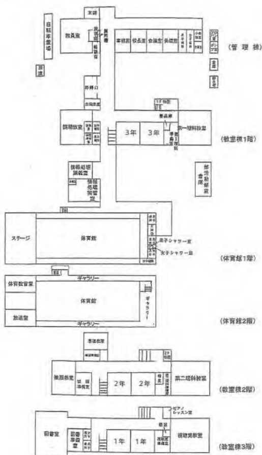
校舎平面図
