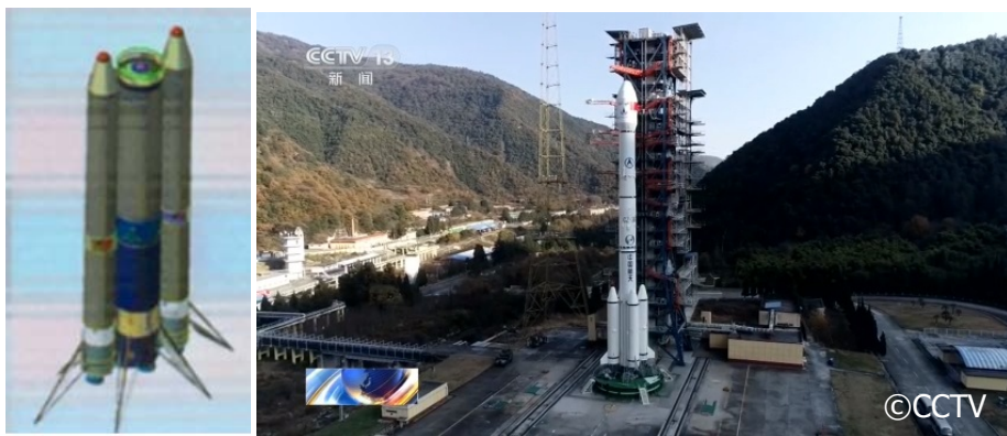
長征8号の1段再使用化の検討例と開発中の長征8号
