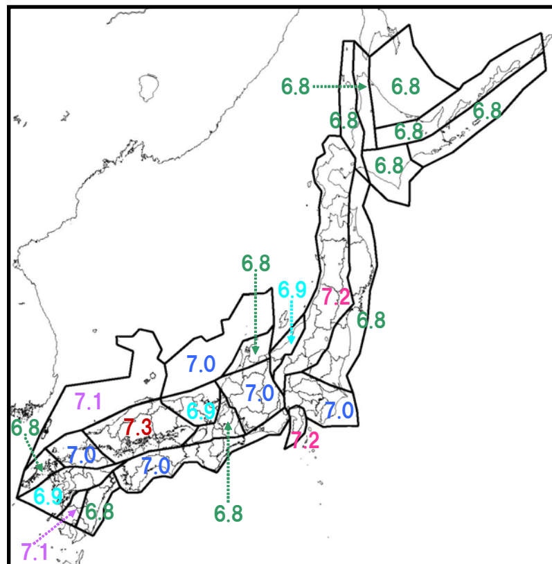
図 2-10 陸域の震源断層を予め特定しにくい地震の最大マグニチュード
