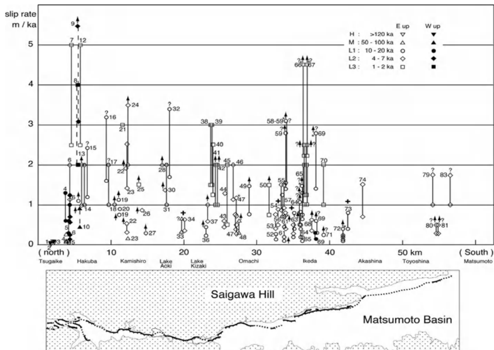
図3-8 糸魚川－静岡構造線断層帯における平均変位速度分布(澤ほか, 2006)
