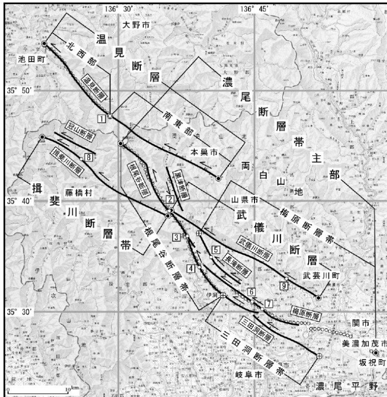
図2-7 複数の単位区間が連動して活動した例(1891 年濃尾地震)
