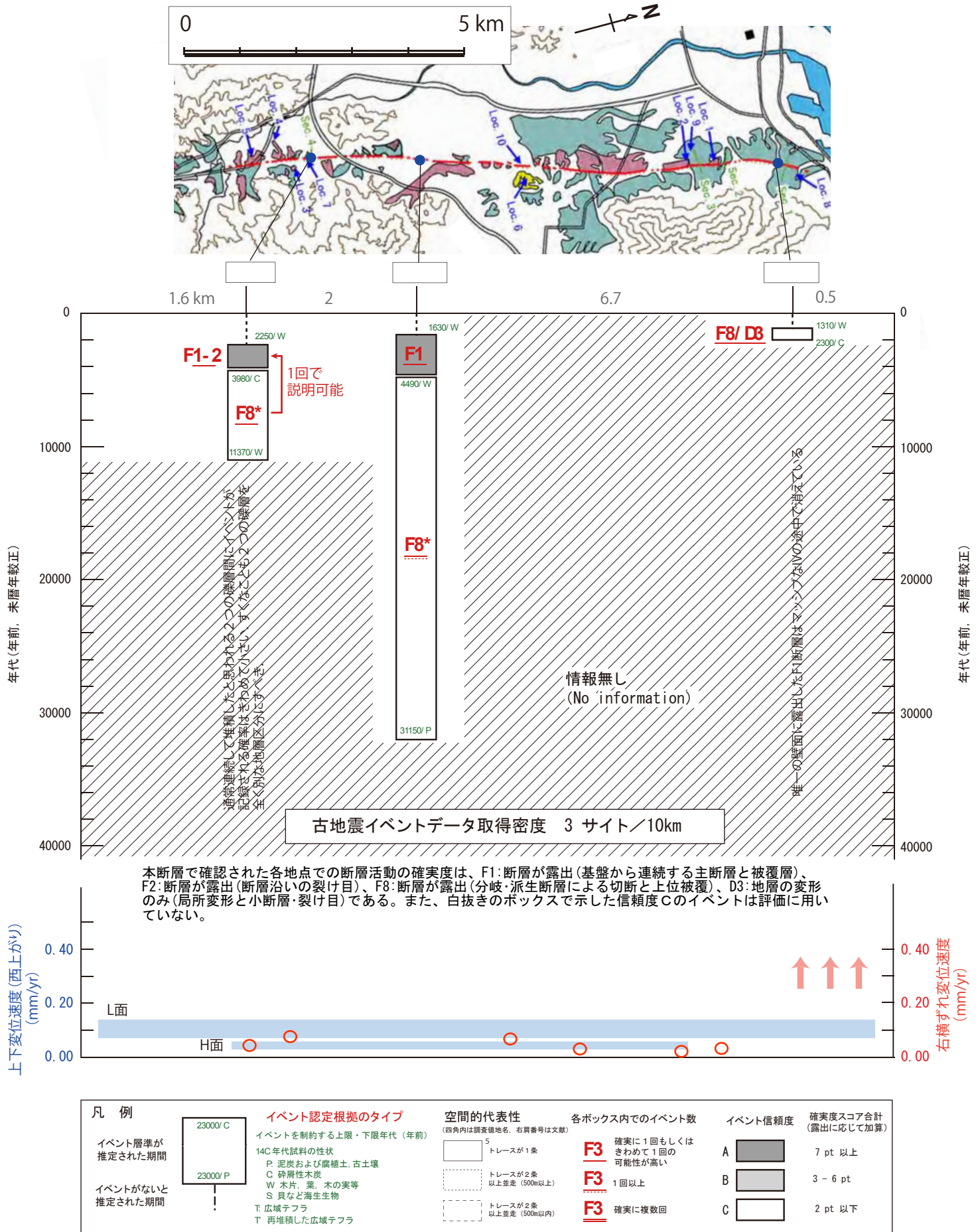
図 2-5 各調査地点における活動時期認定の信頼度を示した時空間ダイアグラムの例
