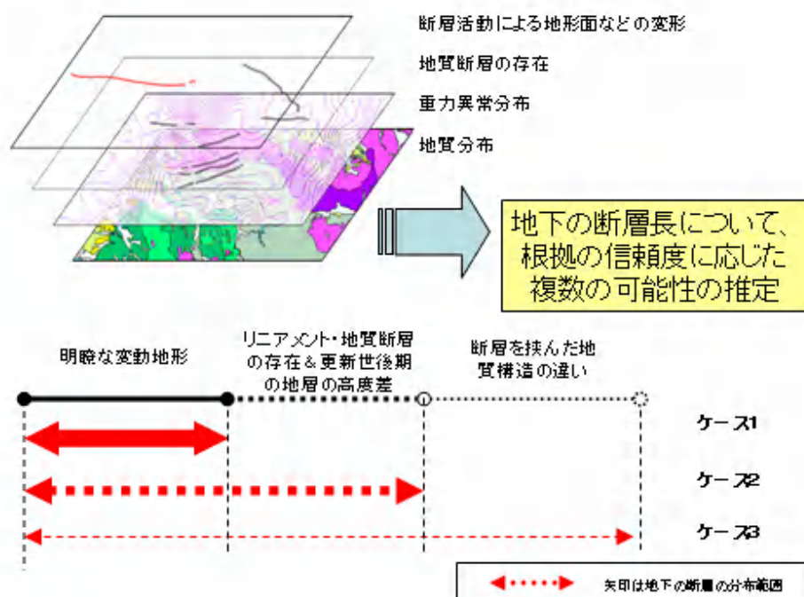
図3-2 地表における長さが「短い活断層」における地下の断層の長さ評価の模式図
