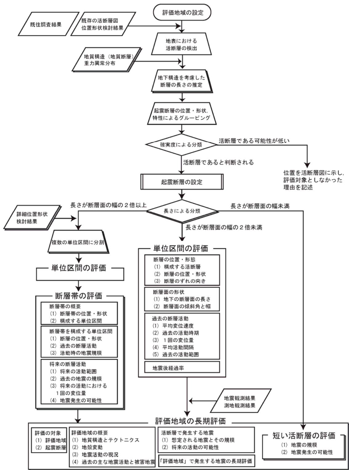
図3-5 評価地域における活断層から発生する地震の長期評価の流れ
