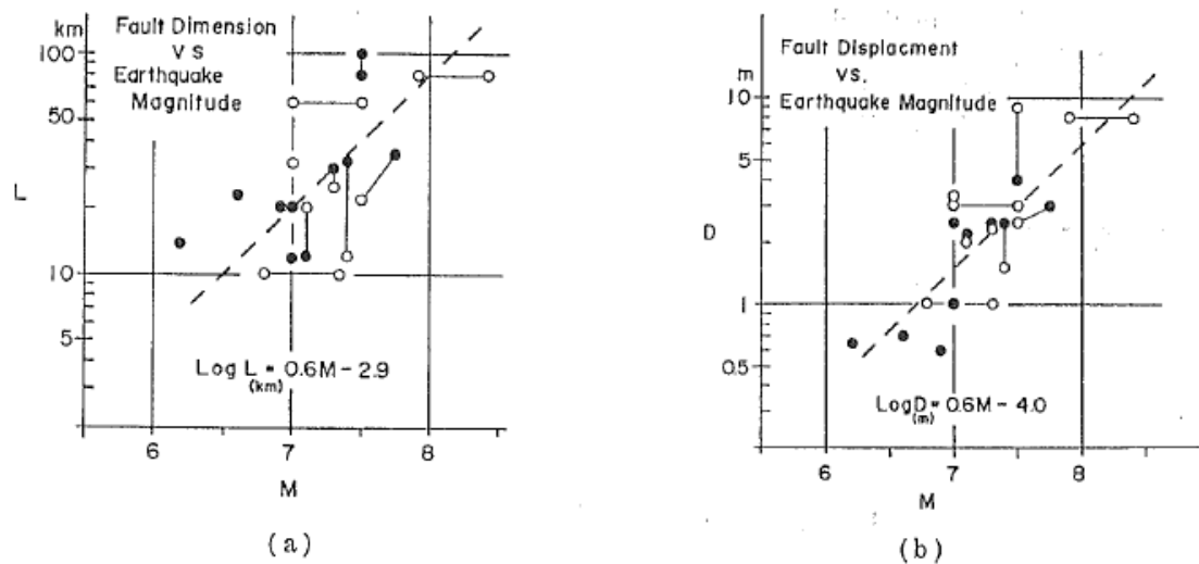
図2-8 地震の規模と、断層の長さ(a)及び地震時のずれ量(b)との関係式(松田, 1975)
