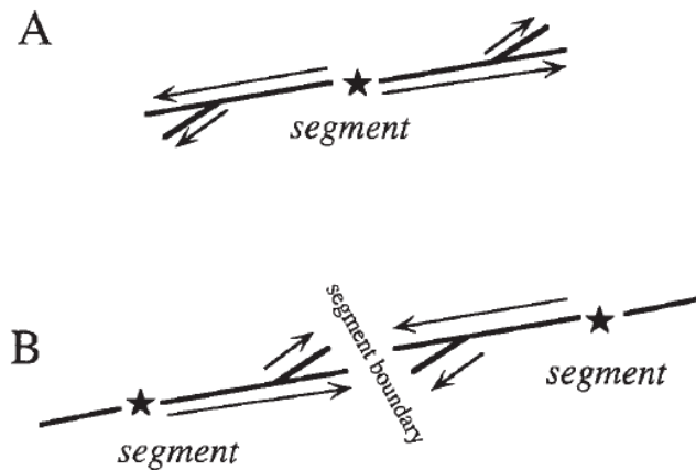
図2-3 断層の分岐形態とセグメント(中田・後藤, 1998)
