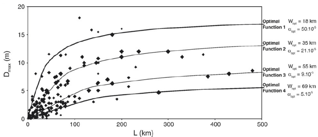
図2-9 長大な断層の事例を含む地表地震断層の長さ地震時のずれ量の関係。記号の大きさは精度を表す。D-L の関係は、断層の成熟度により異なり、すべり量が飽和する長さでいくつかの群に区分される(Manighetti et al , 2007)。
