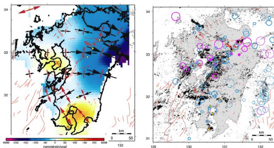
図2ー1 九州におけるひずみ速度(Sagiya, 2004)と応力軸の向きの分布(左)および微小地震活動(気象庁一元化震源を使用)と宇佐美(2003)による歴史地震の分布の比較(右)(検討分科会資料より抜粋)
