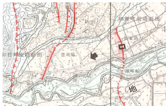
図3-7 変形帯の幅を示した断層線の表現方法の例 都市圏活断層図「北上」(今泉ほか, 2002)
