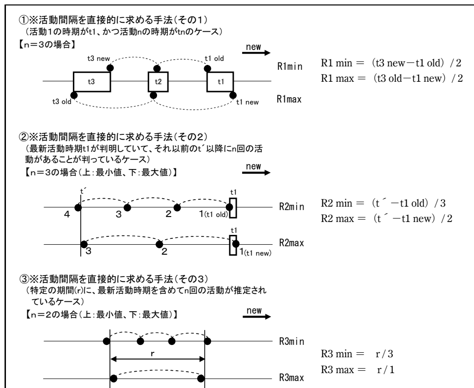
図3-10 直接的手法による平均活動間隔の求め方
