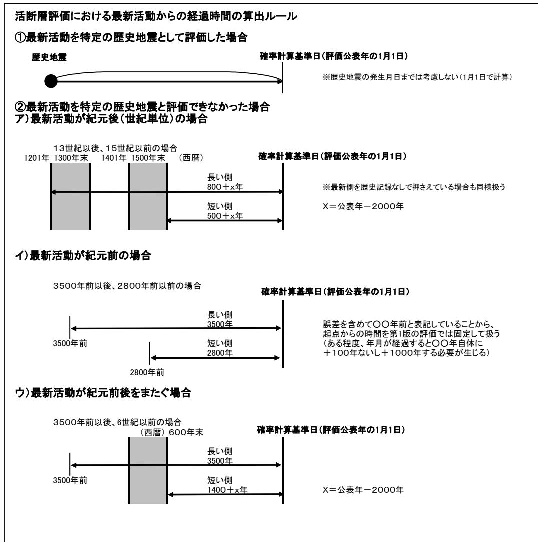
図3-11 最新活動からの経過時間の算出ルール
