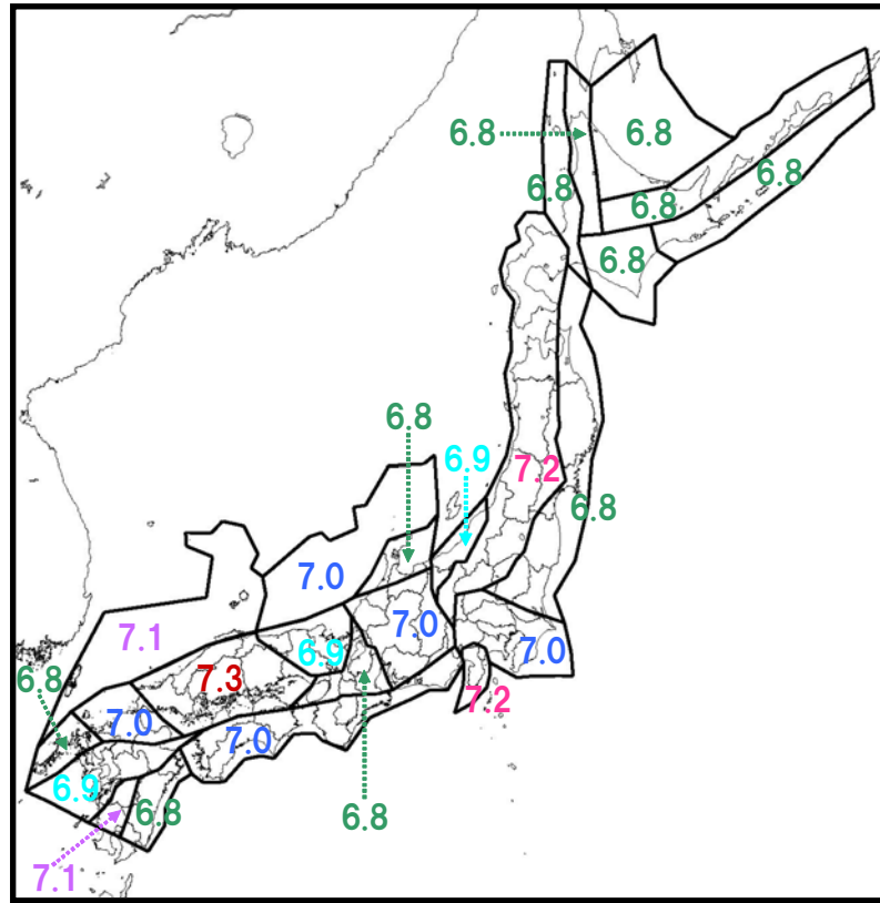
図3-12 陸域の震源断層を予め特定しにくい地震の最大マグニチュード
