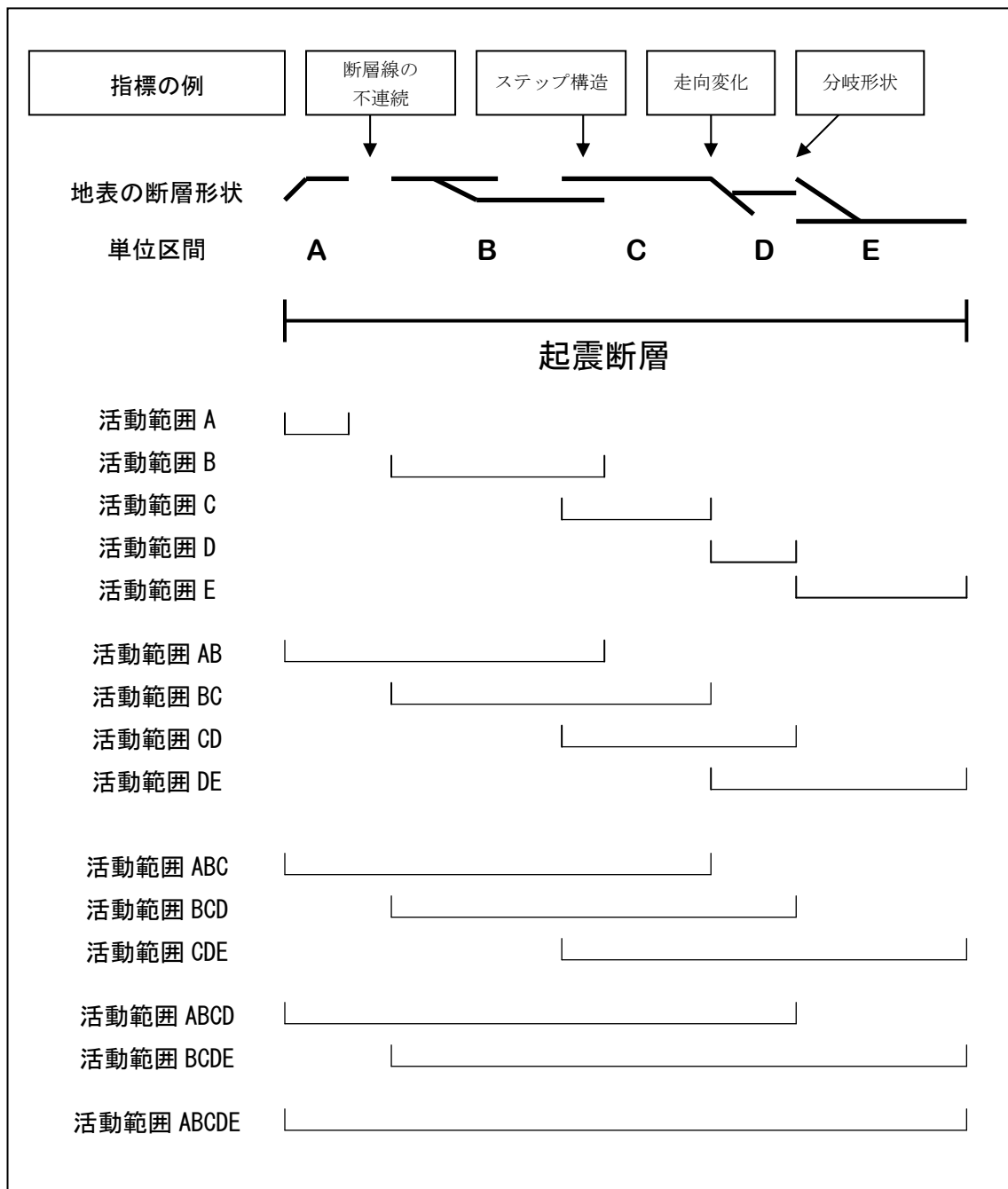
図 3－3 起震断層・活動範囲・単位区間の概念図と起震断層分割の指標の例
