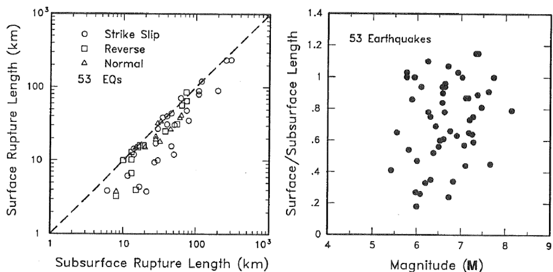
図2-2 地表地震断層と地下の断層の長さの比較(左)と地震規模別にみたそれらの比(右)(Wells and Coppersmith, 1994)
