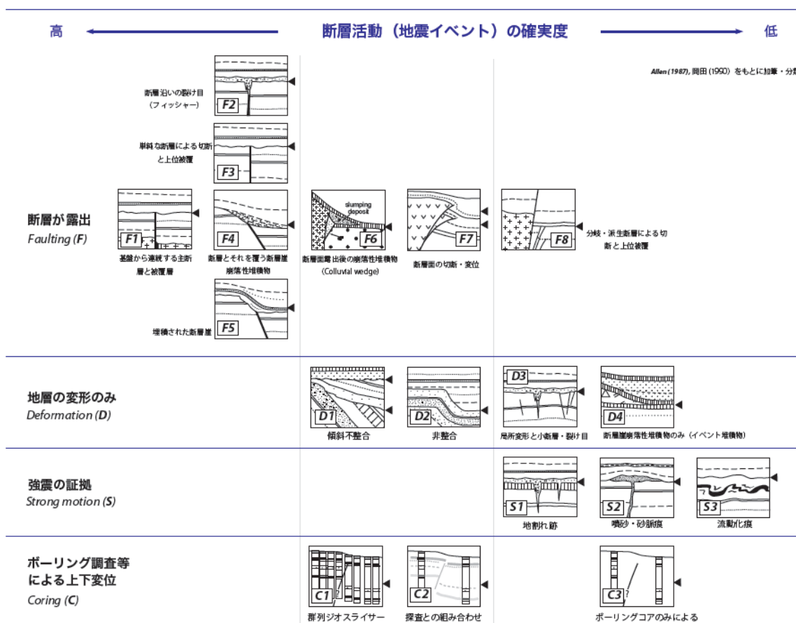
図2-4 地層の変形構造の種類の違いに基づく断層活動の確実度
