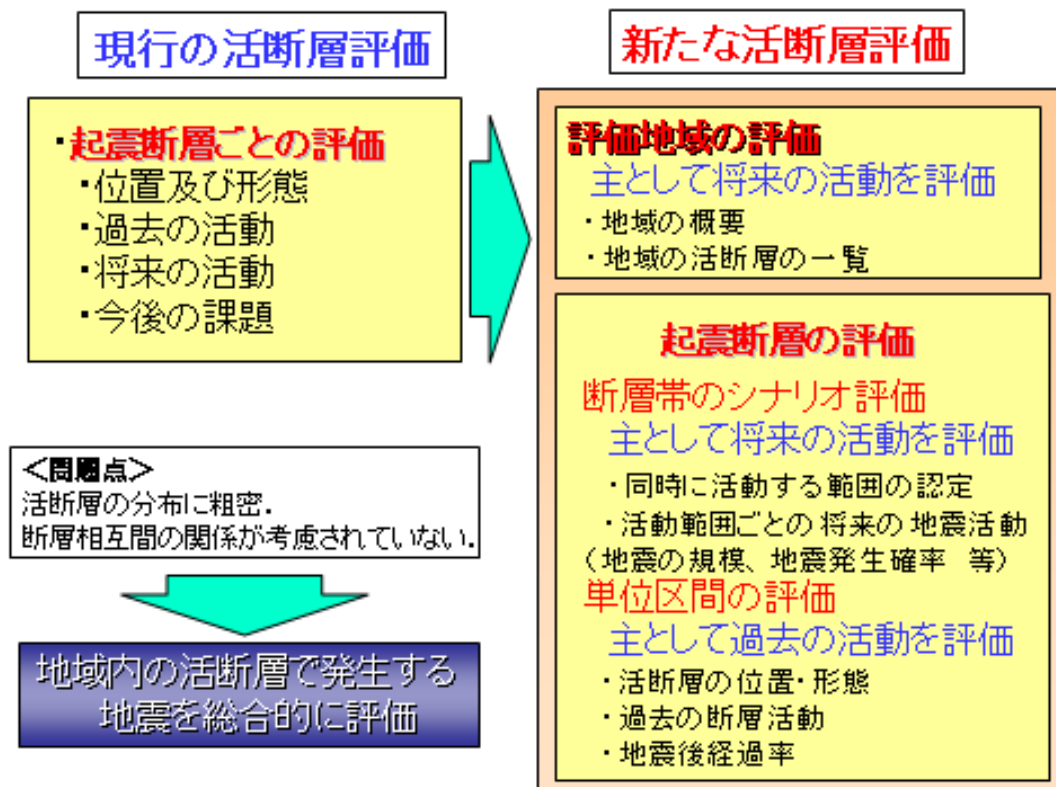
図3-1 これまでの活断層評価の枠組み(左)と新たな活断層評価の枠組み(右)
