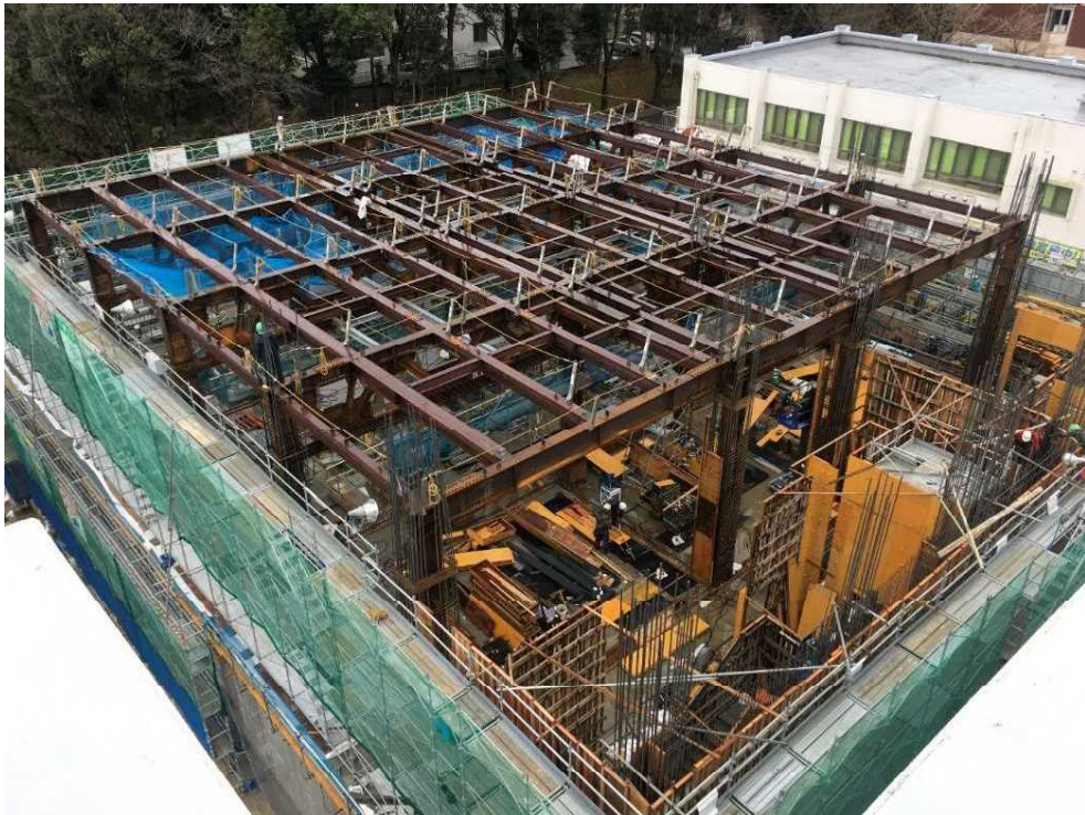
施工状況(全景)
