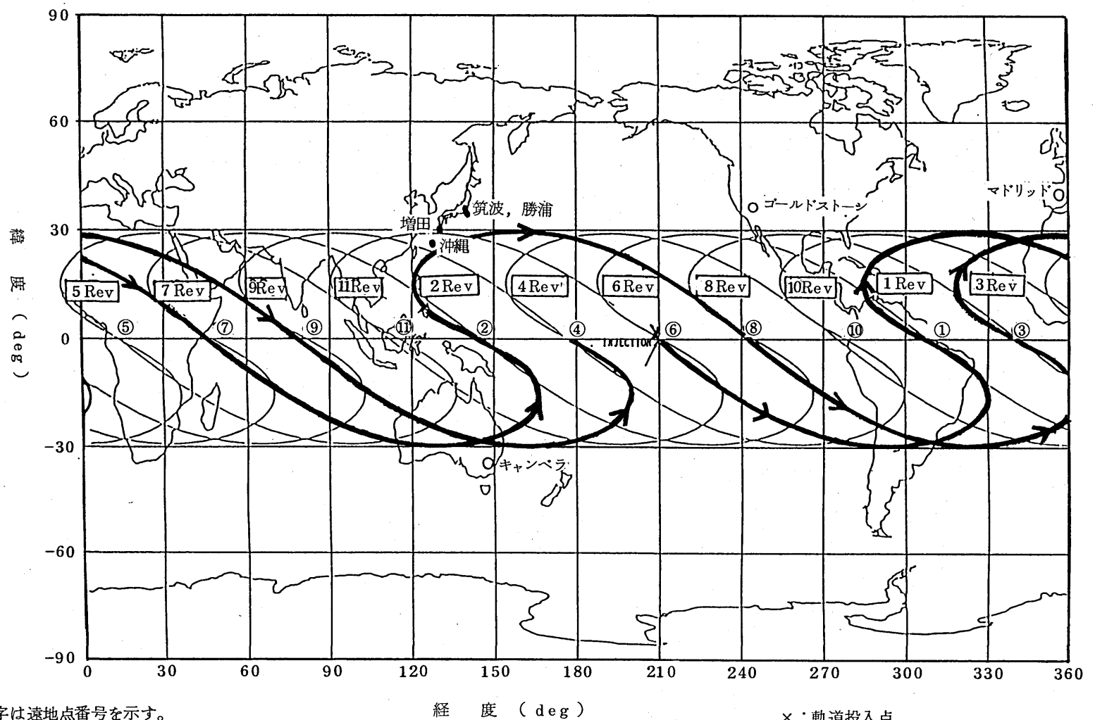
第9図 衛星の地表面軌跡 (トランスファ軌道軌跡)
