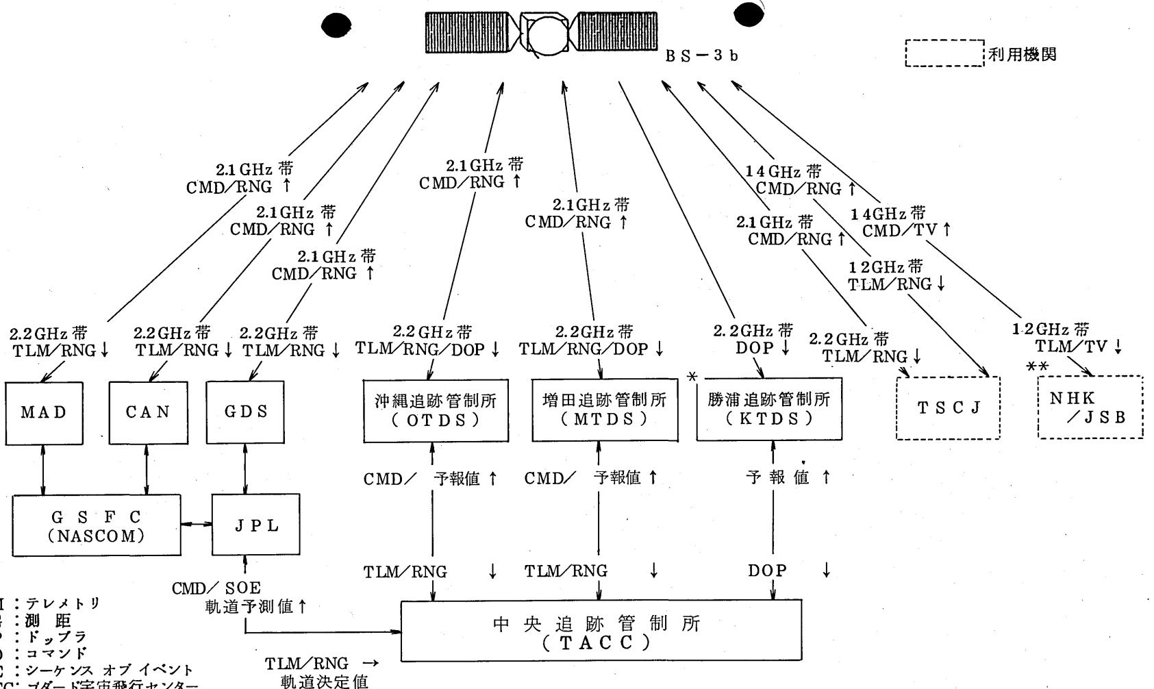
第10図 追跡管制システム (打上げ時及び初期段階)
